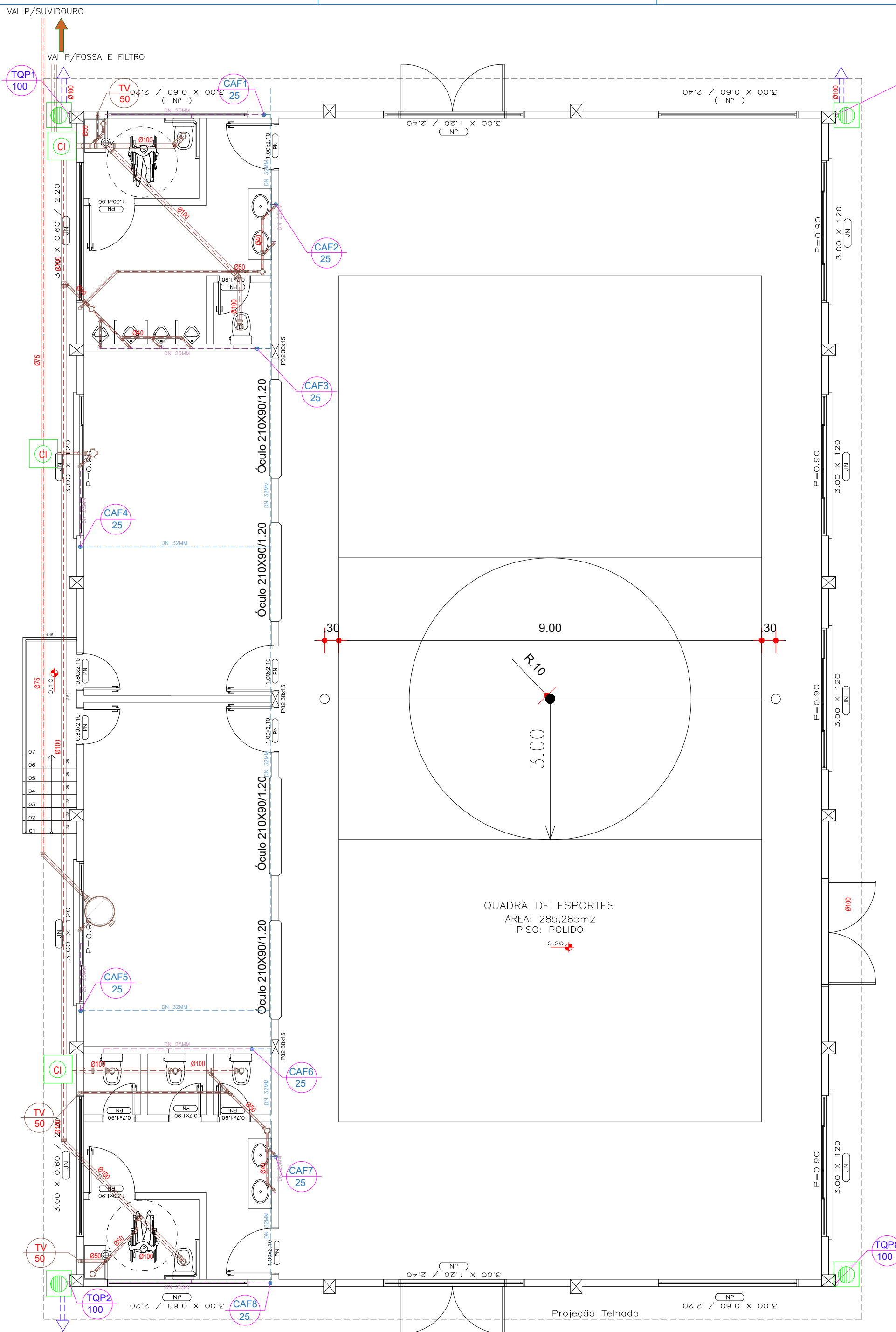
12 HIDROSSANITÁRIO ESCALA: 1/50
