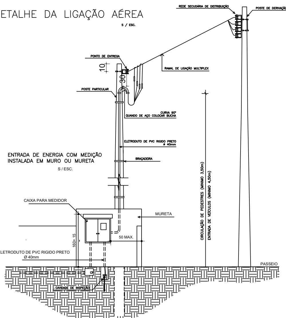
DETALHE DA LIGAÇÃO AÉREA
