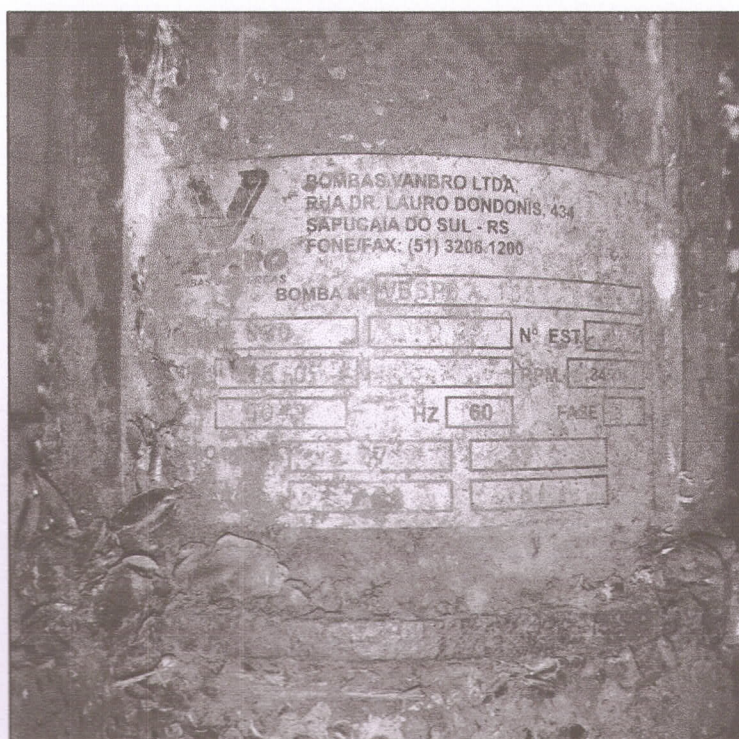
FIGURA 2 – PLACA DE IDENTIFICAÇÃO DO EQUIPAMENTO
