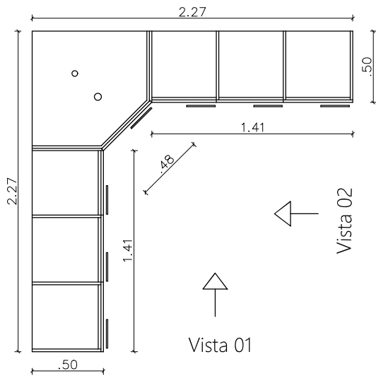
Vista superior sem tampão
