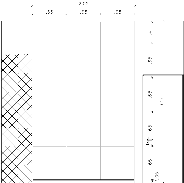
Vista Frontal, sem portas
