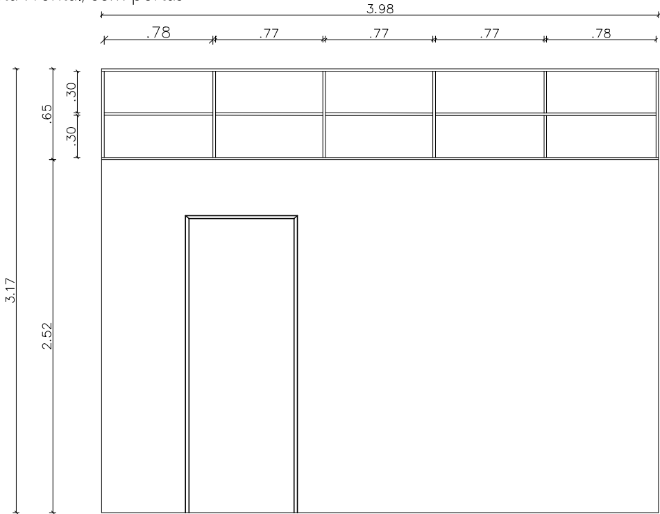
Vista Frontal, sem portas
