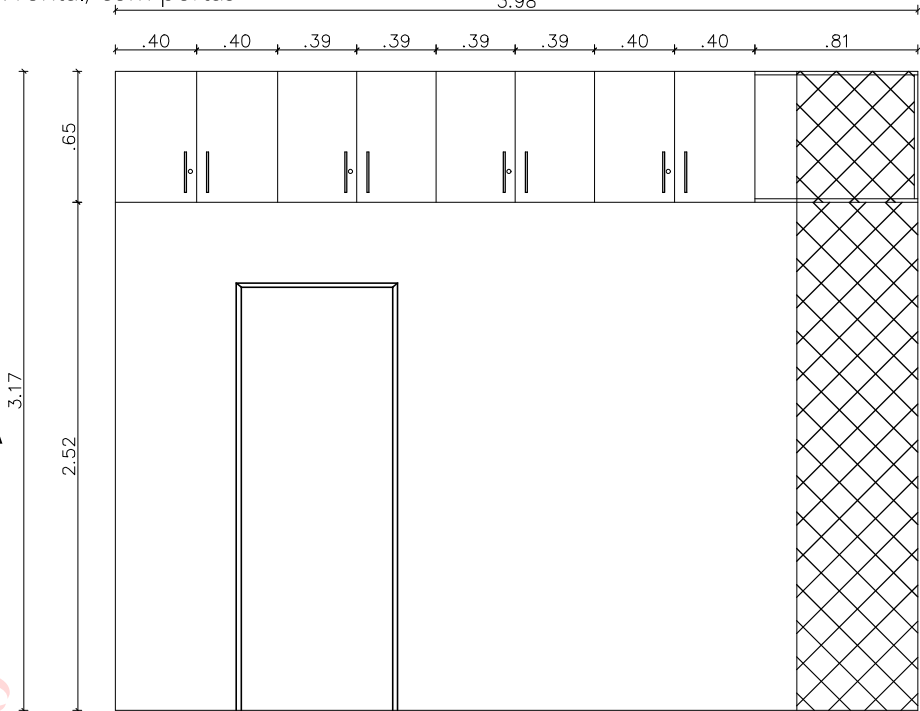
Vista Frontal, com portas
