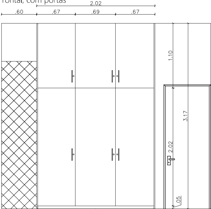
Vista Frontal, com portas
