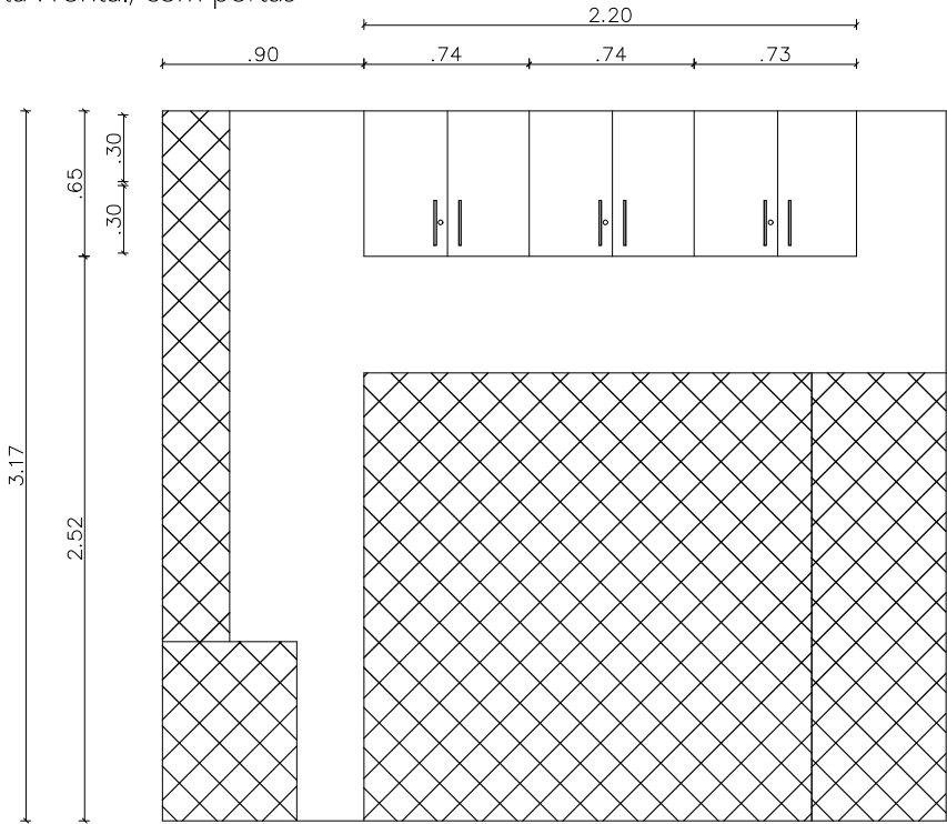
Vista Frontal, com portas
