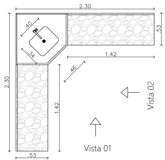
Vista superior com tampão
