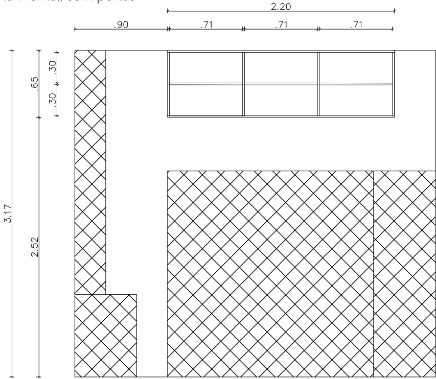
Vista Frontal, sem portas
