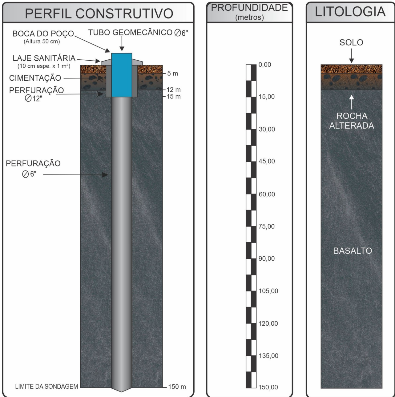
Figura 1. Perfil geológico e projeto construtivo básico do poço tubular.
