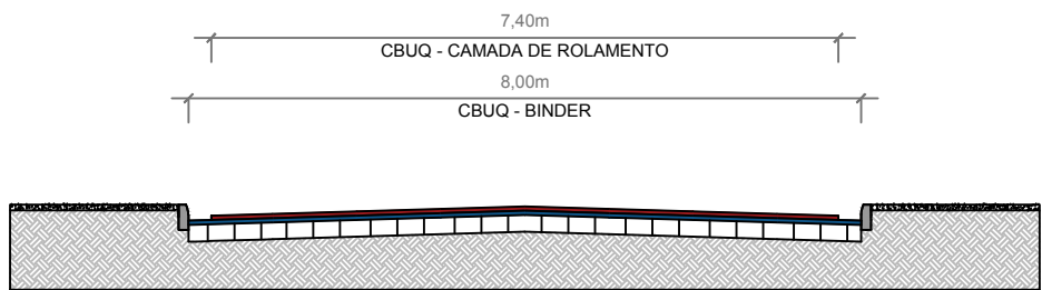
SEÇÃO TIPO DE PAVIMENTAÇÃO Sem escala RUA HERCULES PASINATTO
