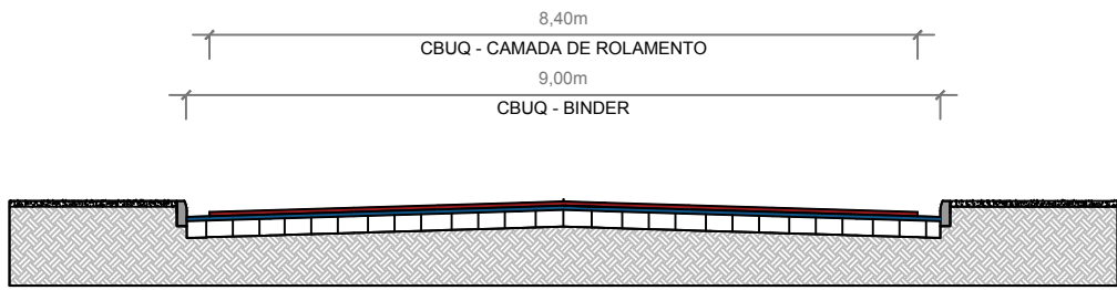
SEÇÃO TIPO DE PAVIMENTAÇÃO Sem escala RUA JOSÉ JUNGES
