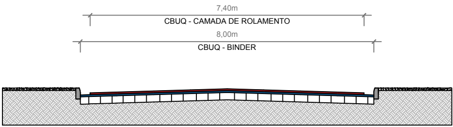
SEÇÃO TIPO DE PAVIMENTAÇÃO Sem escala RUA MAXIMO MORGAM
