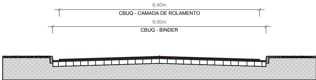
SEÇÃO TIPO DE PAVIMENTAÇÃO Sem escala
