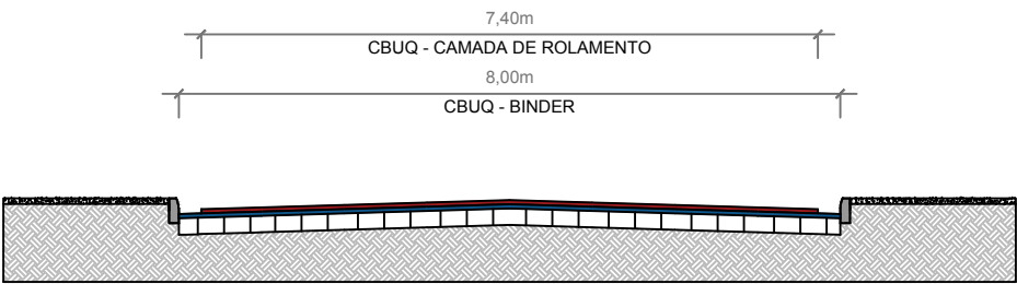
SEÇÃO TIPO DE PAVIMENTAÇÃO Sem escala
