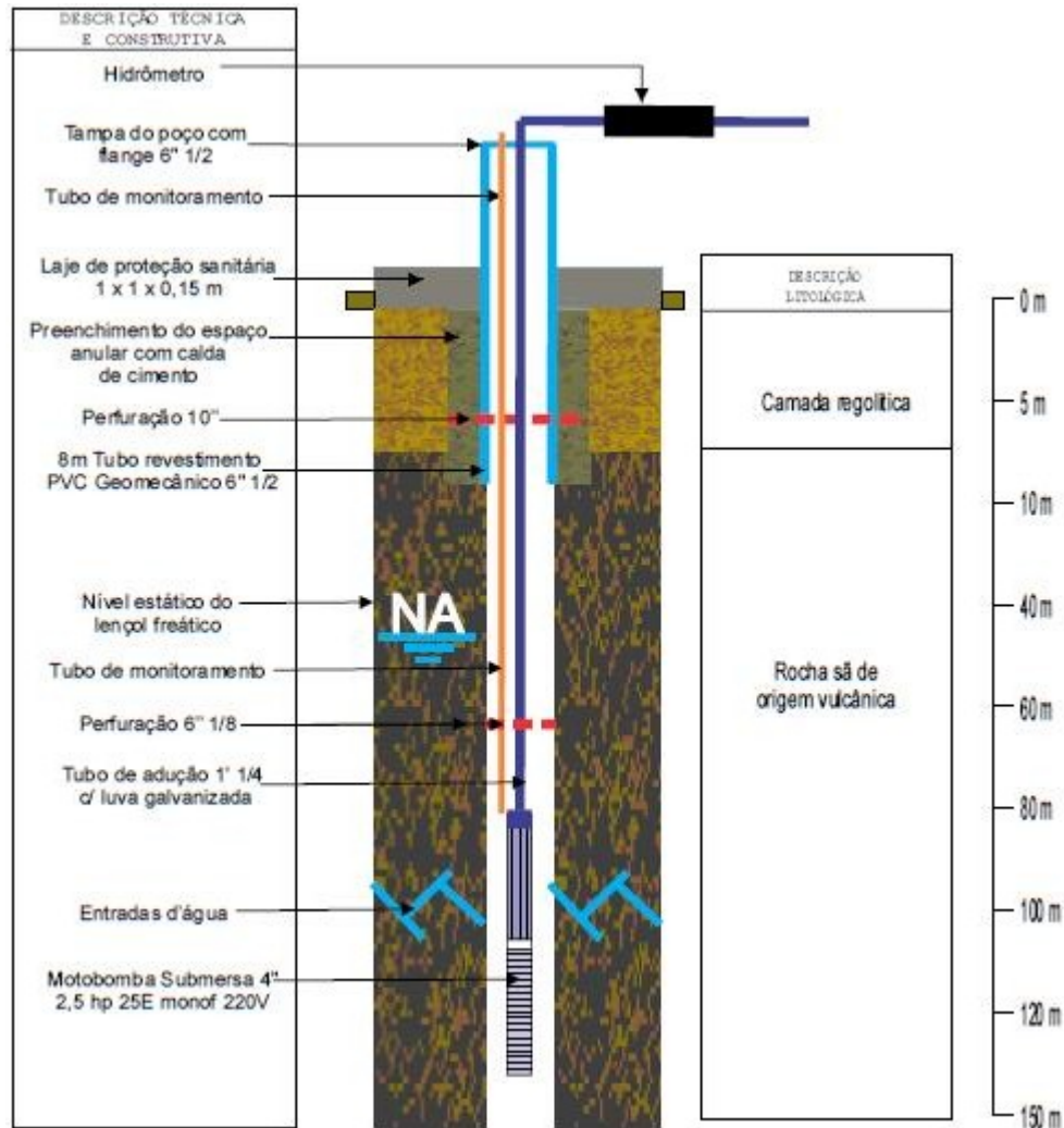
Figura 12: Perfil esquemático de poço tubular profundo.
