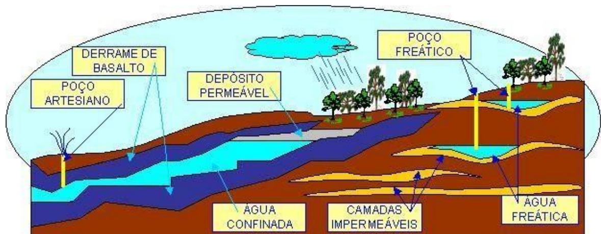
Figura 7: Tipos de poços
