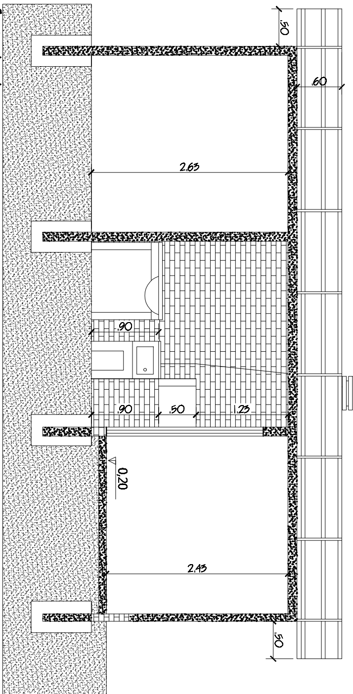
Corte A - A
