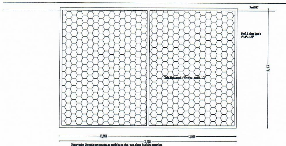
Detalhe do Fechamento com Tela Hexagonal - Esc.: 1: 210
