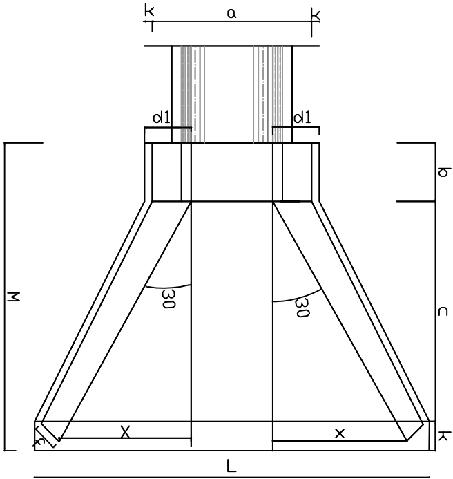
Bueiros Normais
