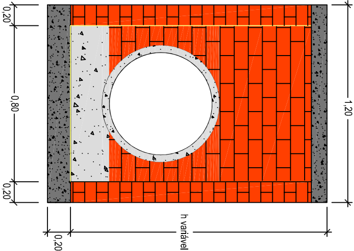
SEÇÃO AA'
