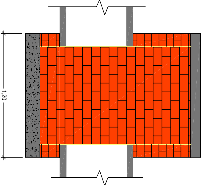
SEÇÃO BB'
