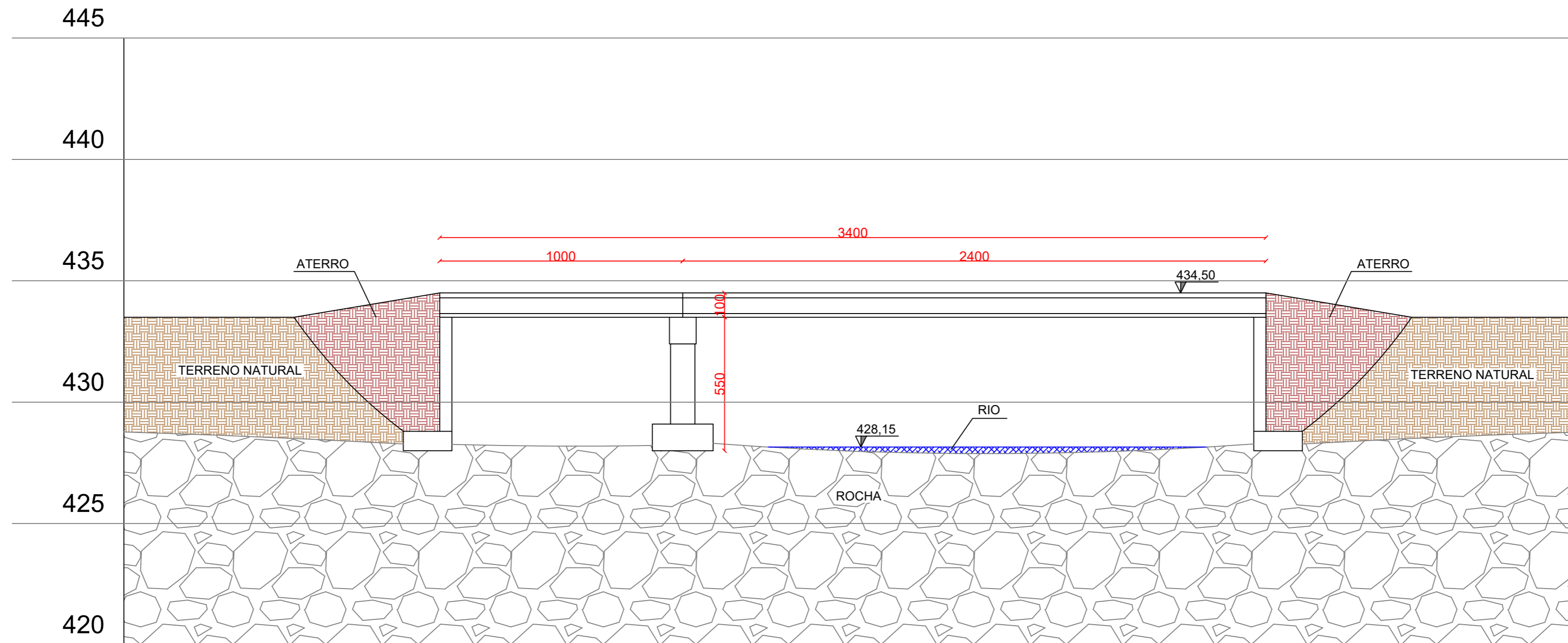
01 SEÇÃO DE CORTE E ATERRO
