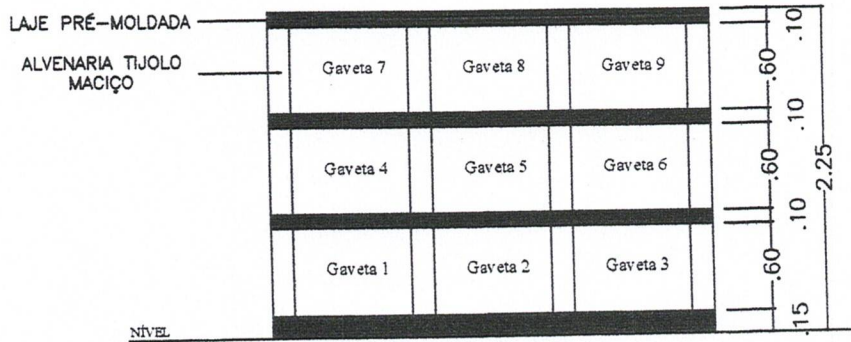
CORTE A-A' ÁREA: 8,4 m 2
