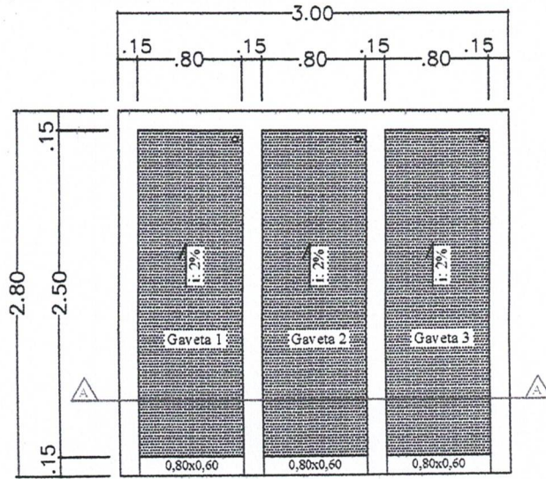
PLANTA BAIXA ÁREA: 8,4 m 2
