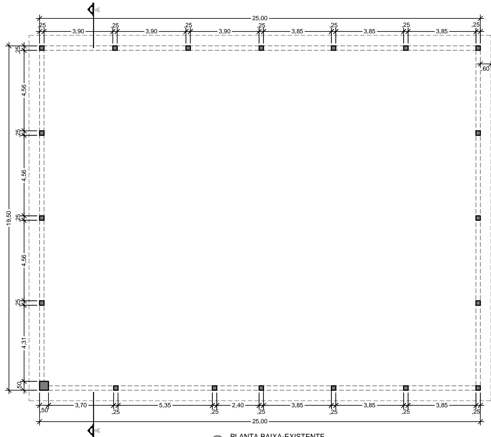
01 PLANTA BAIXA-EXISTENTE ESCALA: 1/100 ÁREA: 487,50m 2
