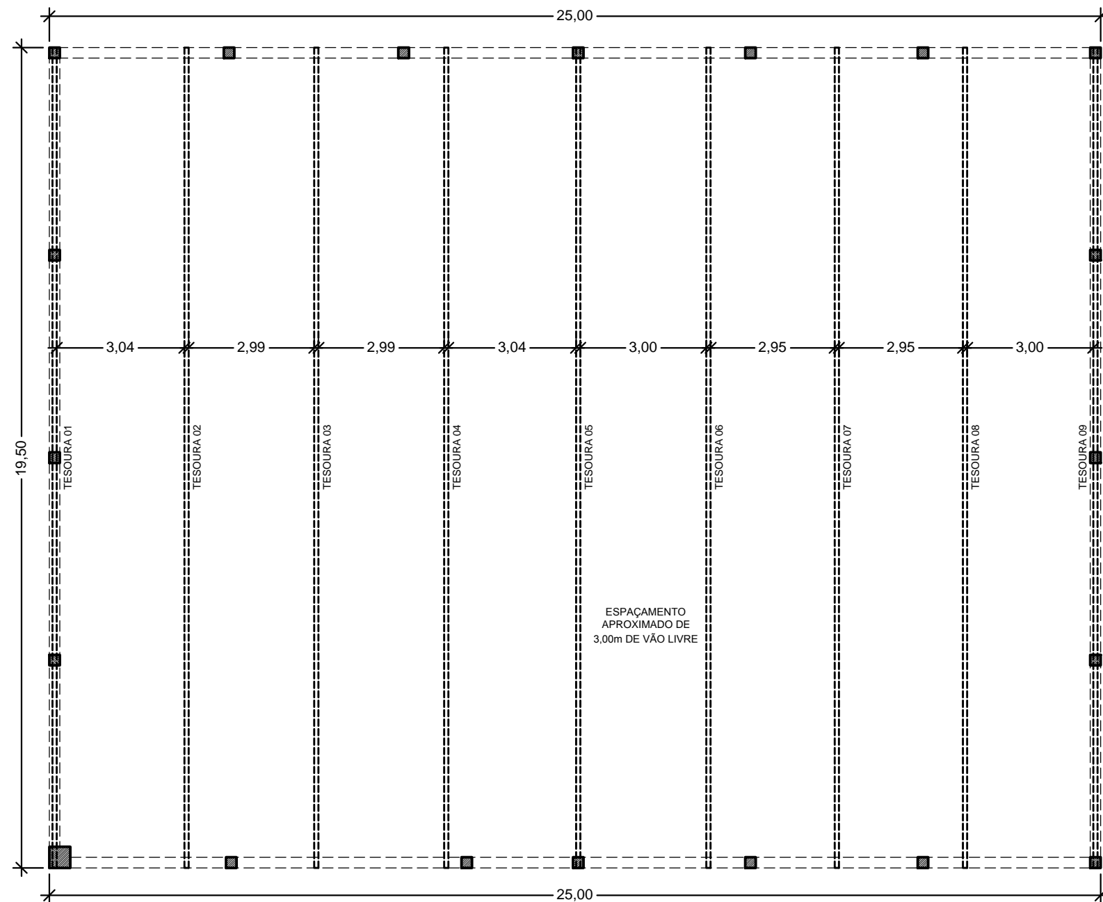
01 POSIÇÃO DAS TESOURAS EXISTENTES ESCALA: 1/100 ÁREA: 487,50m 2
