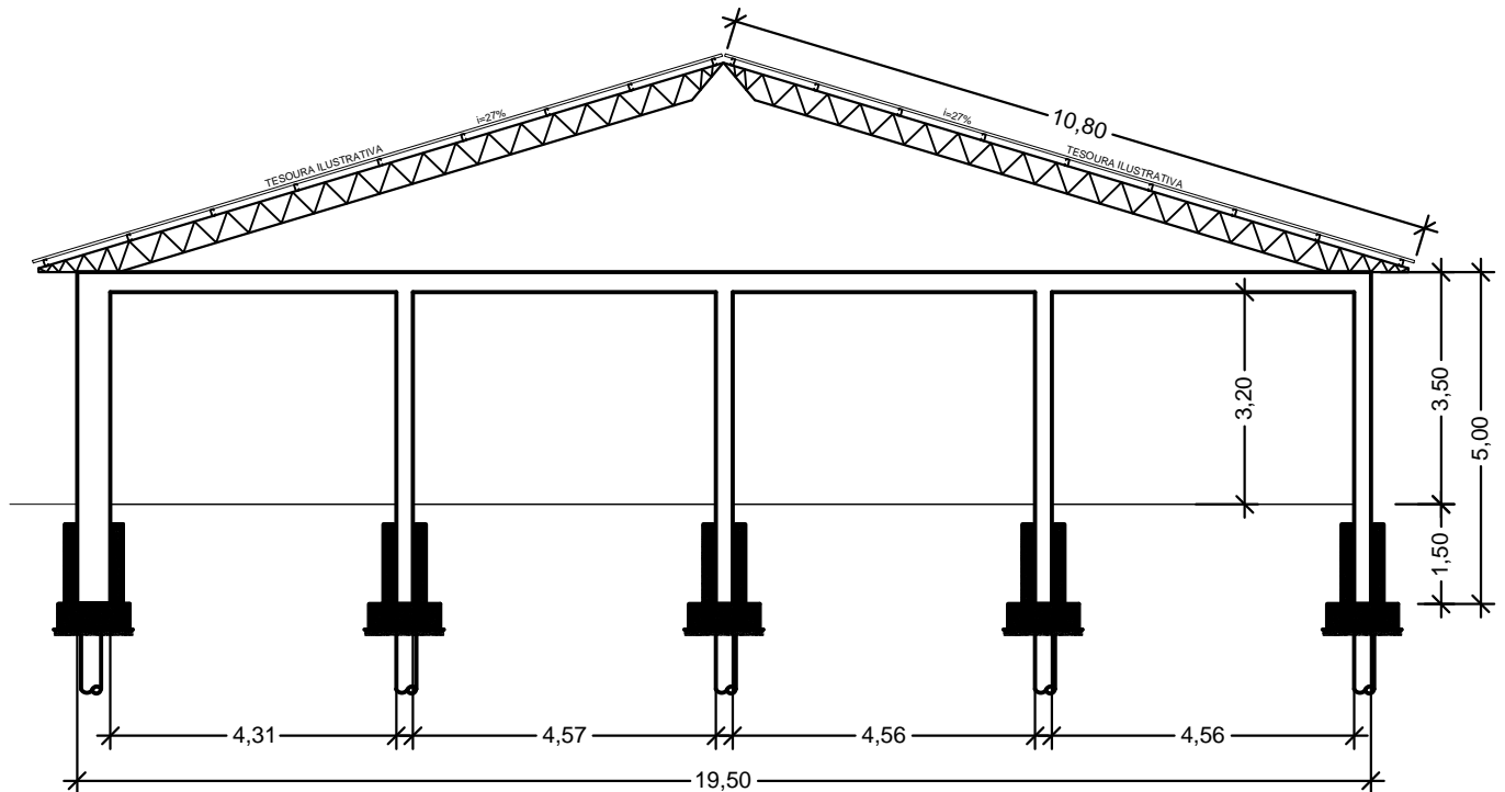
01 CORTE AA ESCALA: 1/100 PARTE EXISTENTE
