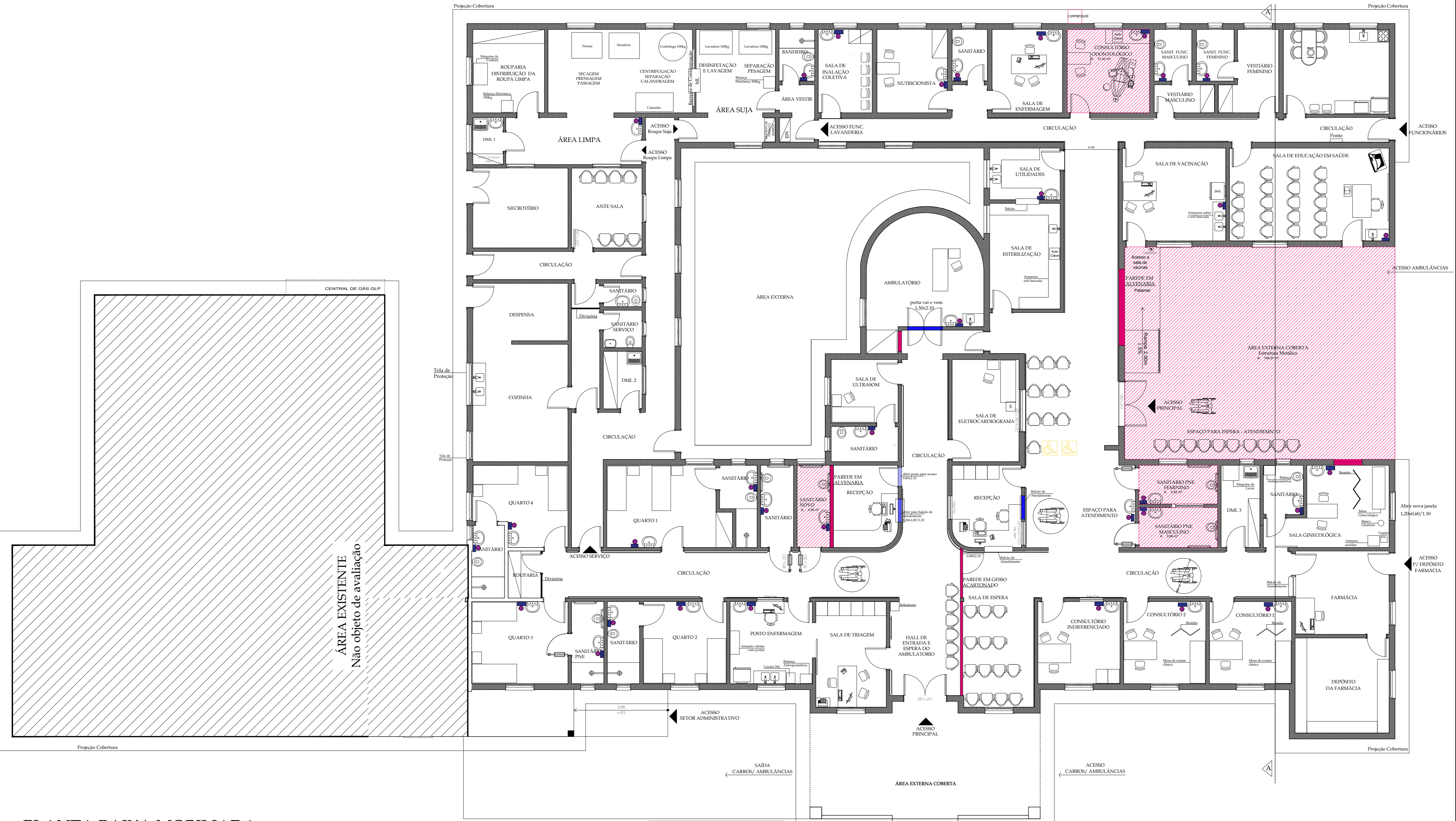
PLANTA BAIXA MOBILIADA Esc.: 1/100
