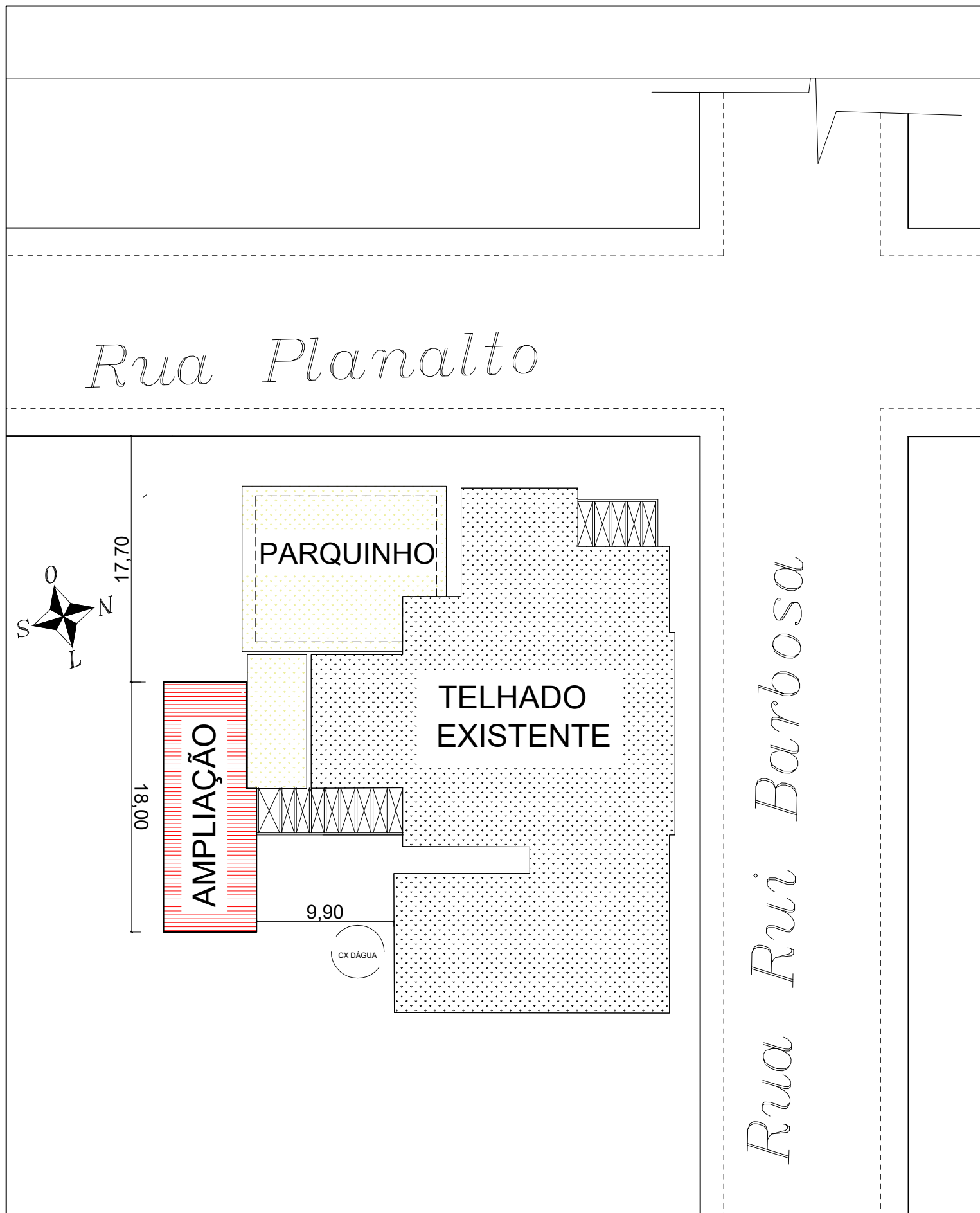
PLANTA DE LOCAÇÃO - ESC.:1/100
