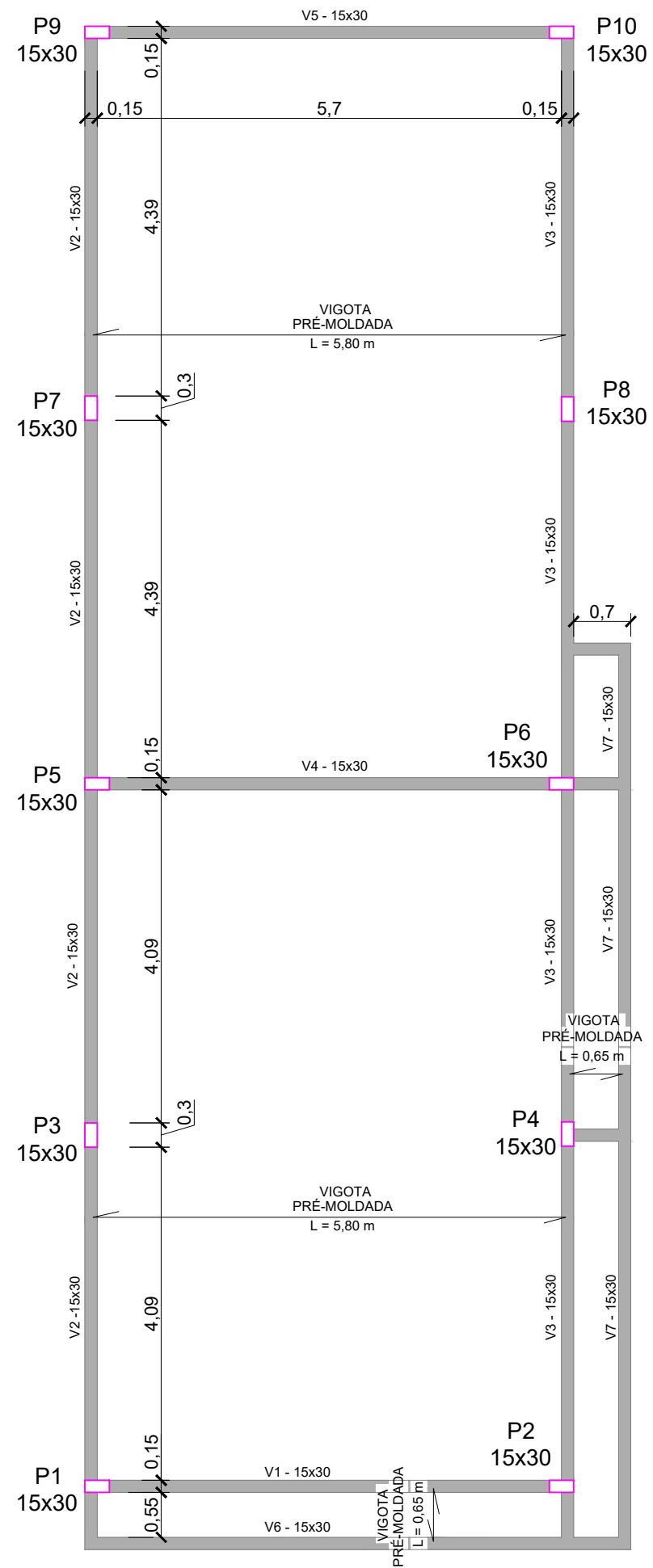
PLANTA DE FORMA DAS VIGAS SUPERIORES ESCALA 1/75
