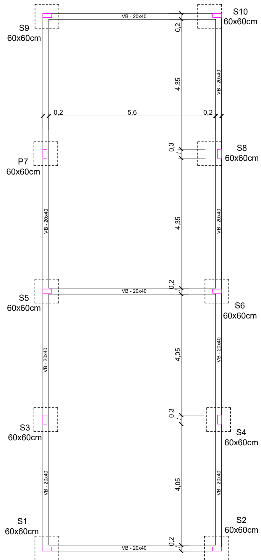
PLANTA DE FORMA DAS VIGAS BALDRAME E LOCALIZAÇÃO DAS SAPATAS - ESCALA 1/75
