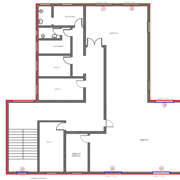
PLANTA BAIXA SEGUNDO PAVIMENTO Esc.: 1/200
