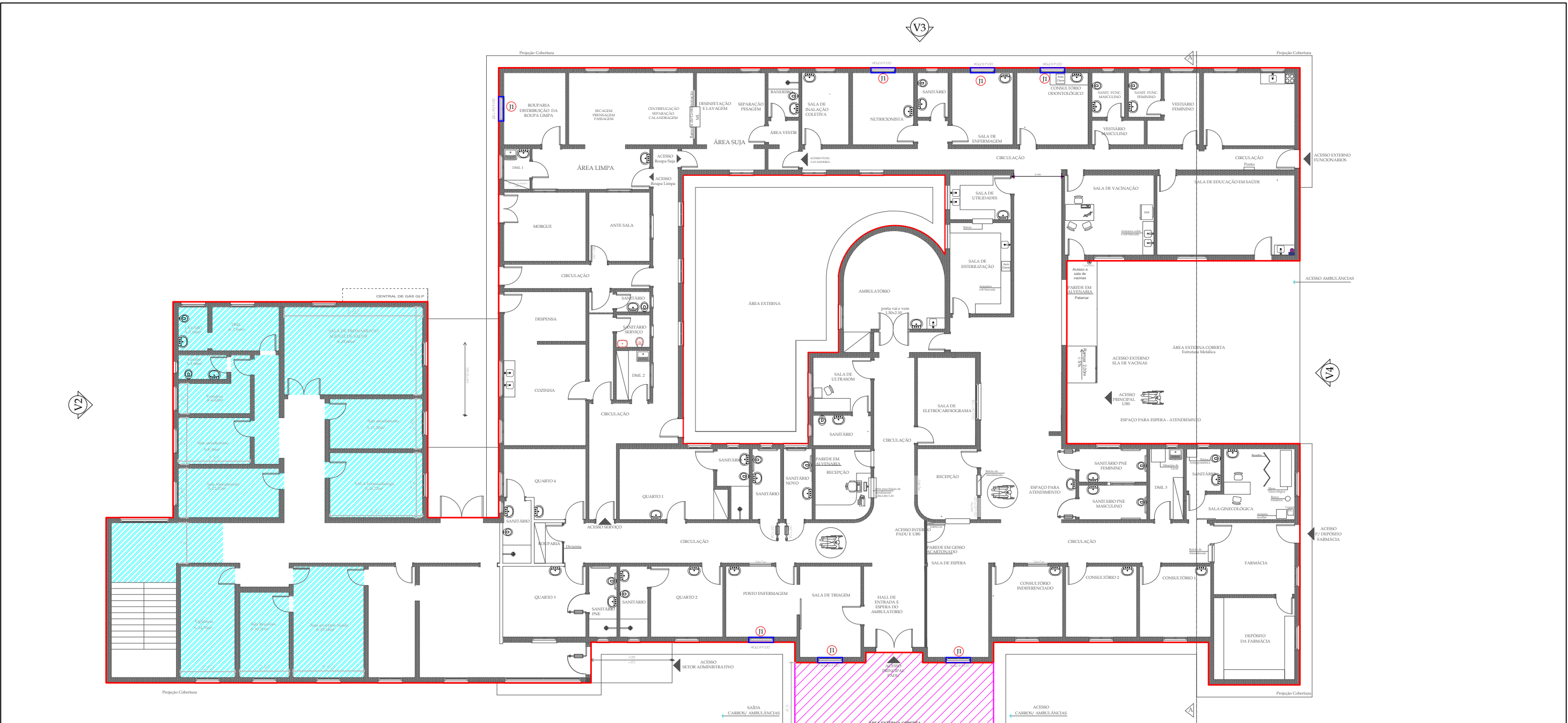
PLANTA BAIXA MOBILIADA Esc.: 1/100
