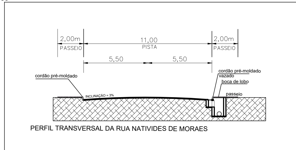
PERFIL TRANSVERSAL SEM ESCALA
