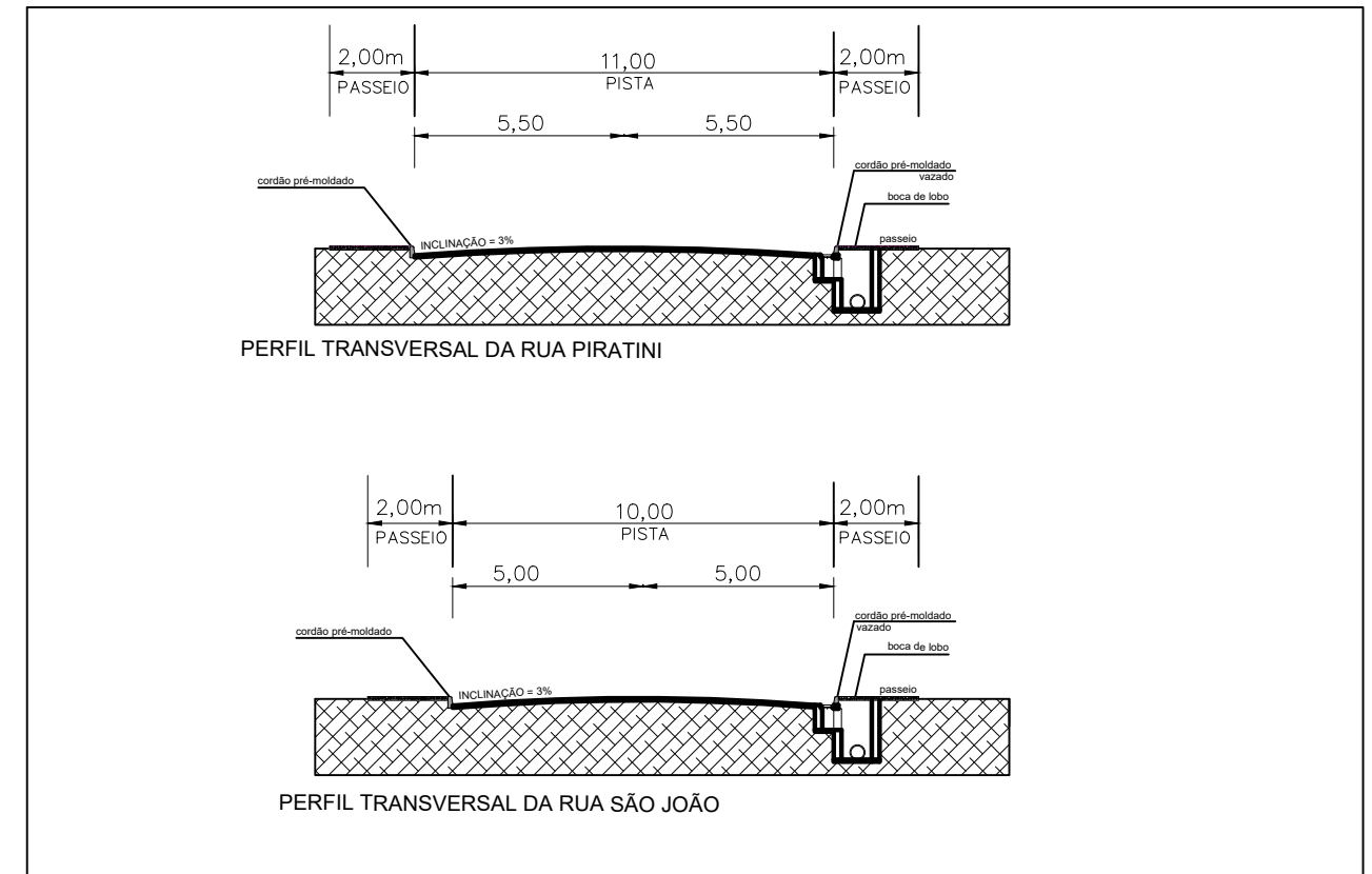
PERFIL TRANSVERSAL S/E
