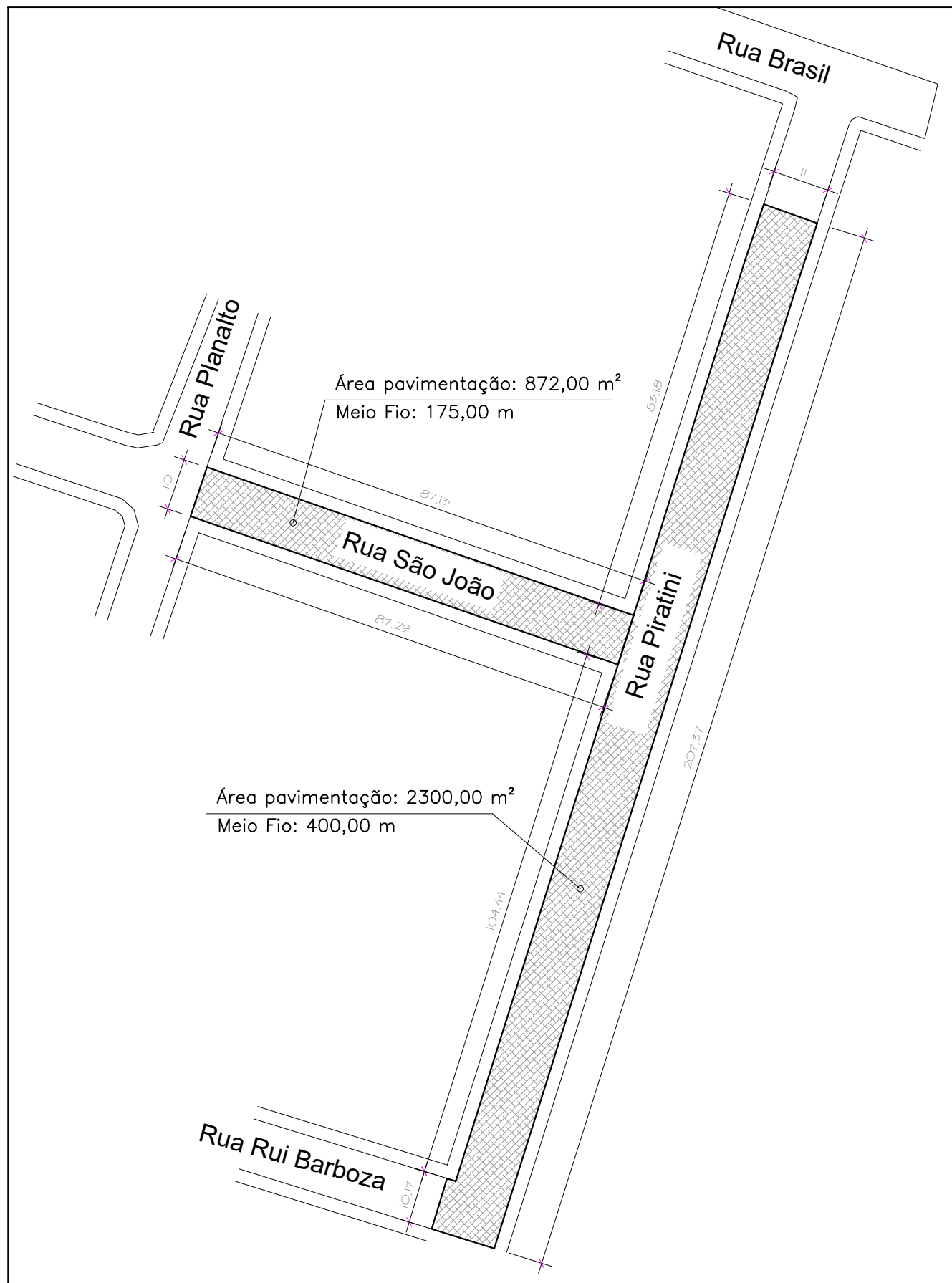
PLANTA BAIXA PAVIMENTAÇÃO - RUA SÃO JOÃO E RUA PIRATINI 1:1000
