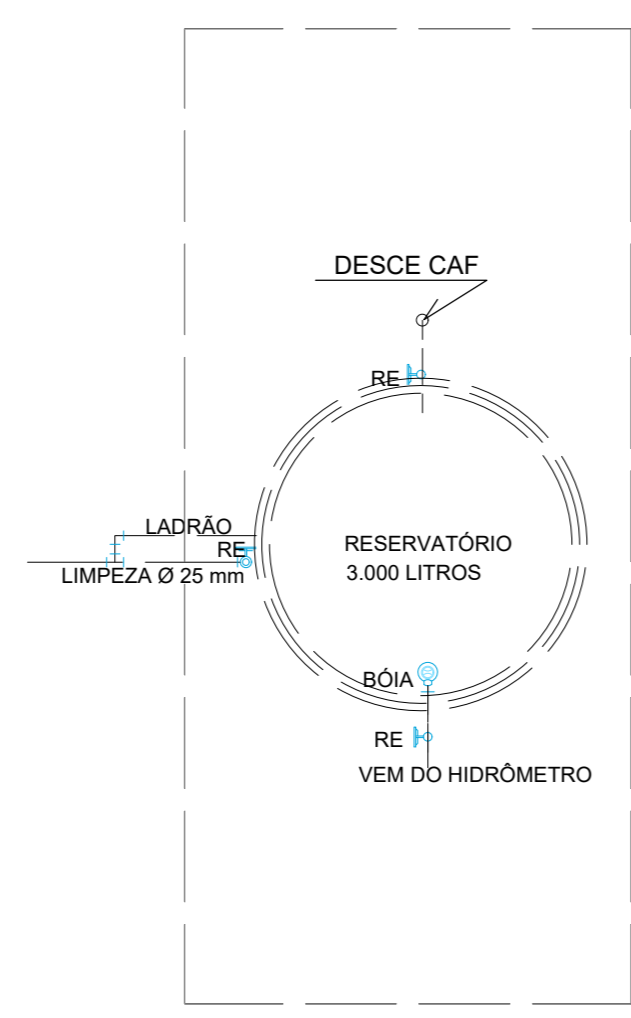
DETALHE 01 BLOCO SOBRE SANITÁRIOS
