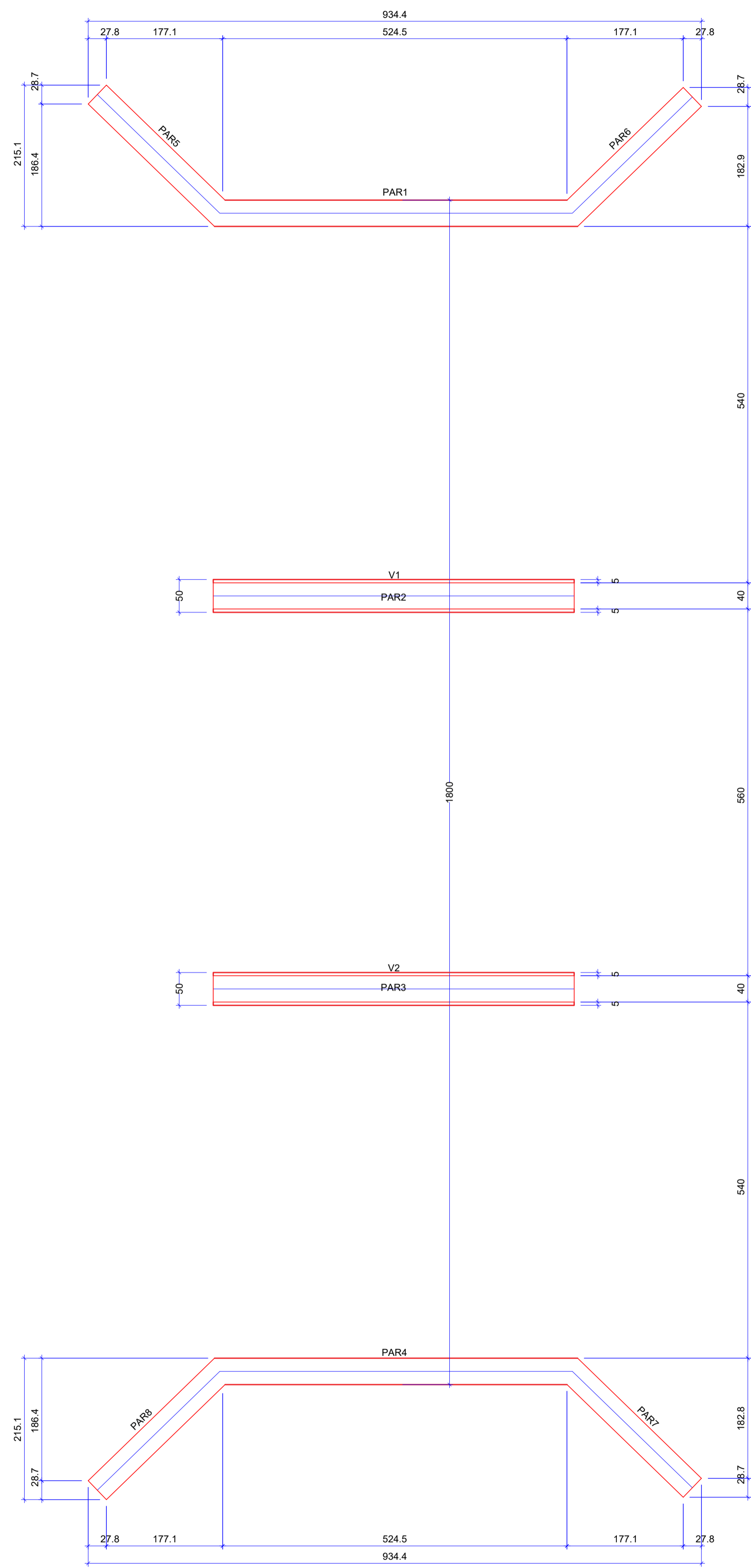
Forma do pavimento Elevação escala 1:50
