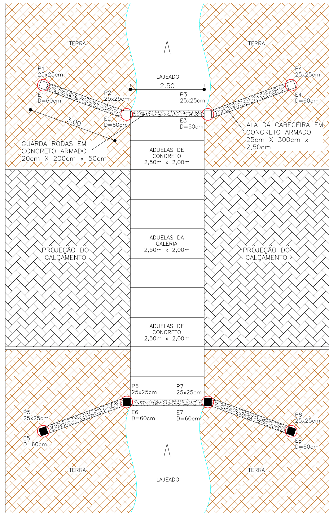
PLANTA BAIXA
