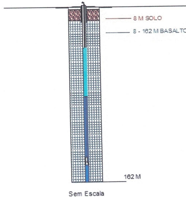
Figura 13: Perfil Geológico do Poço. Fonte: Autor (2024).
