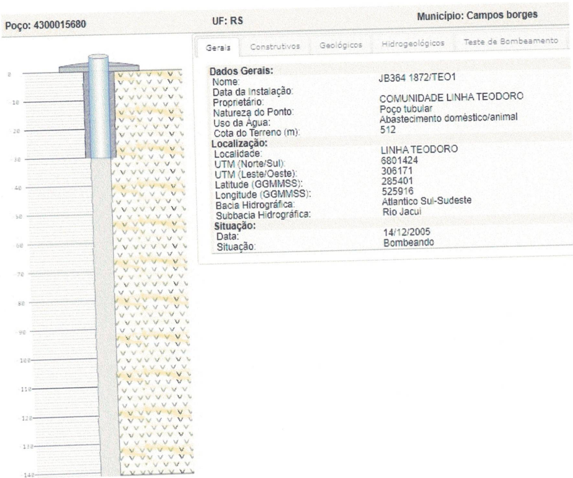
Figura 11: Perfil Geológico do Poço 1. Fonte: SIAGAS (2024).
