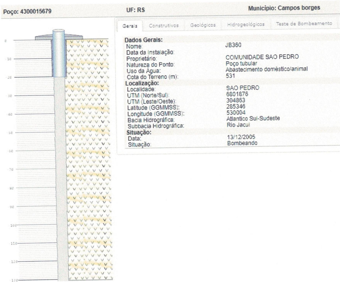
Figura 12: Perfil Geológico do Poço 2. Fonte: SIAGAS (2024).
