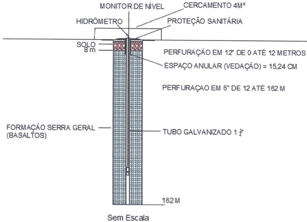
Figura 14: Perfil Construtivo do Poço. Fonte: Autor (2024).
