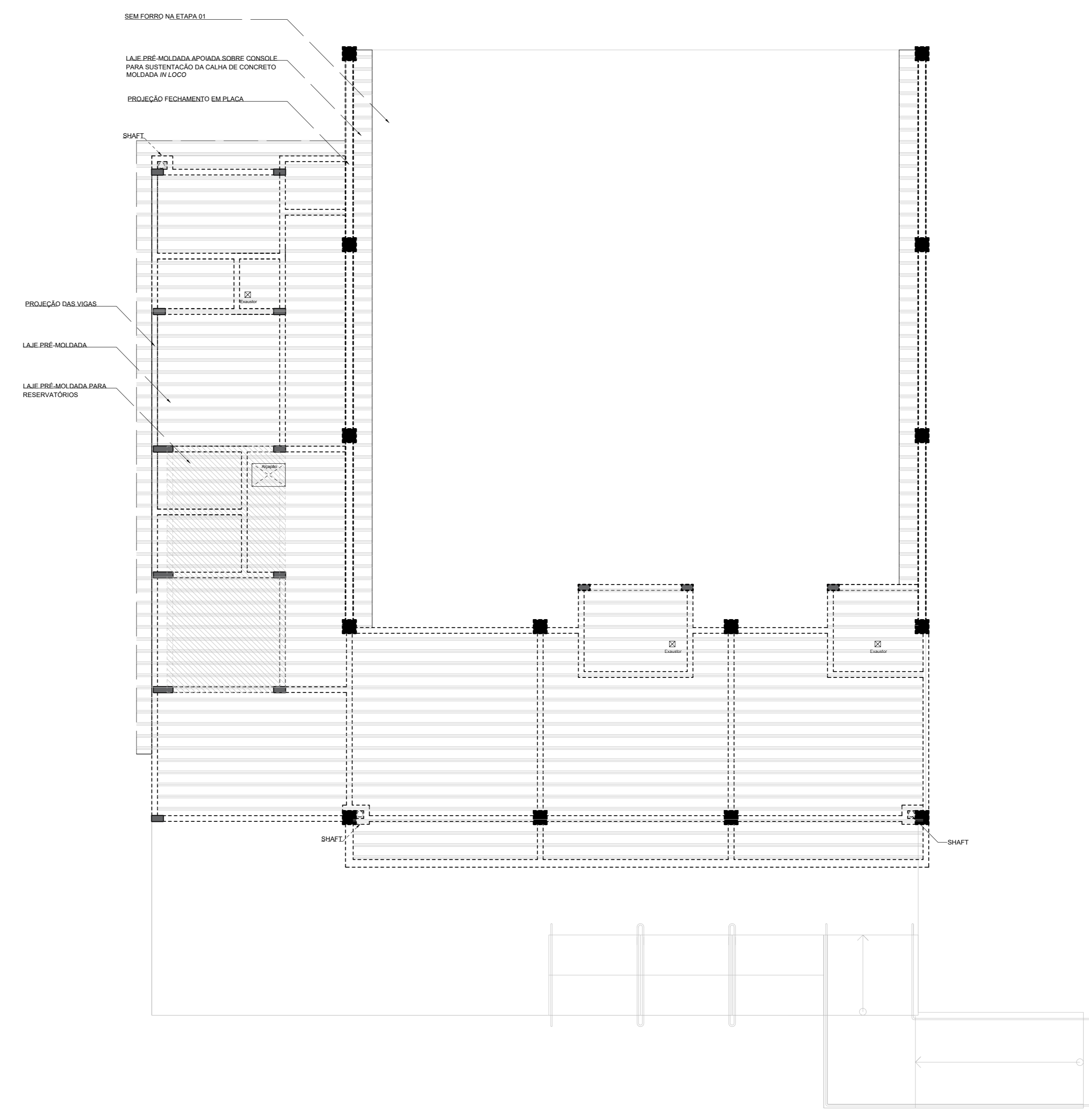
PLANTA DE FORRO 1/75
