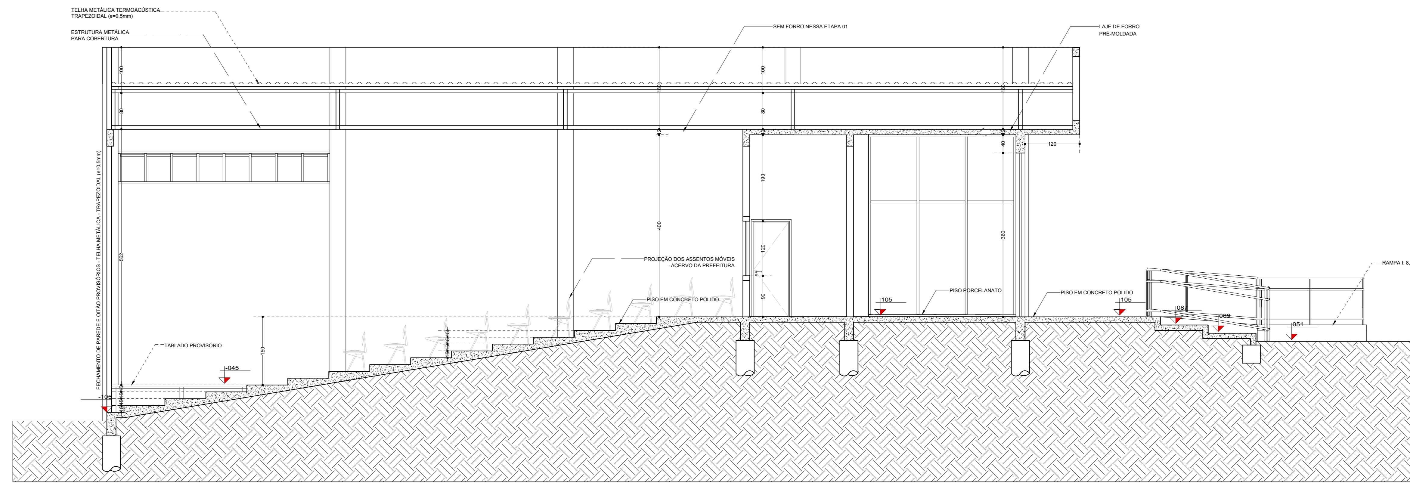
CORTE E - F 1/50
