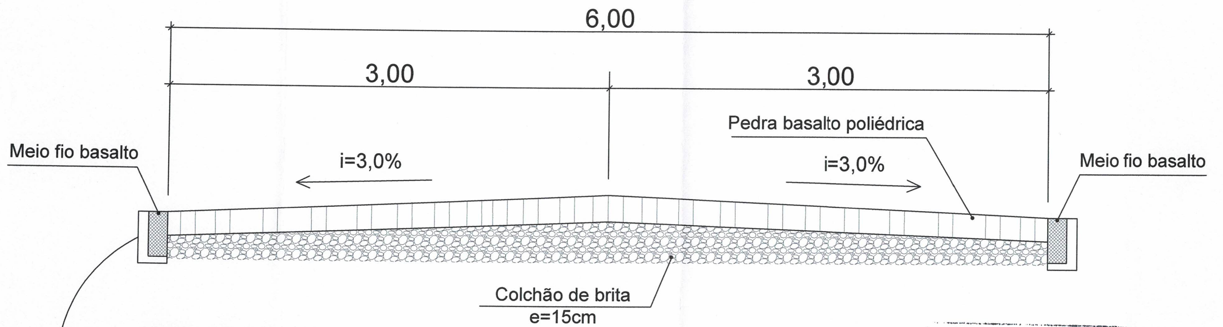
PERFIL TRANSVERSAL ESCALA: 1/25
