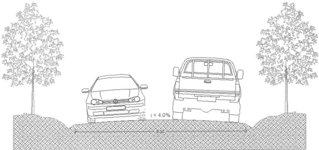
SEÇÃO TRANSVERSAL
