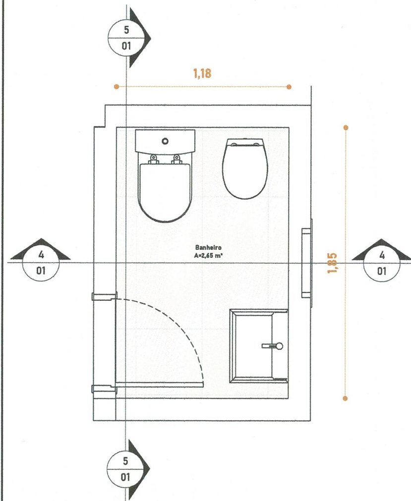
1 Banheiro 1 1:25
