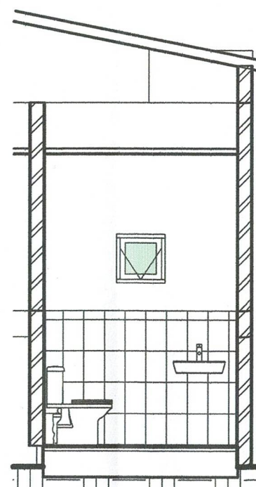
5 Corte 3 1:50
