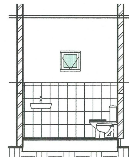
6 Corte 4 1:50
