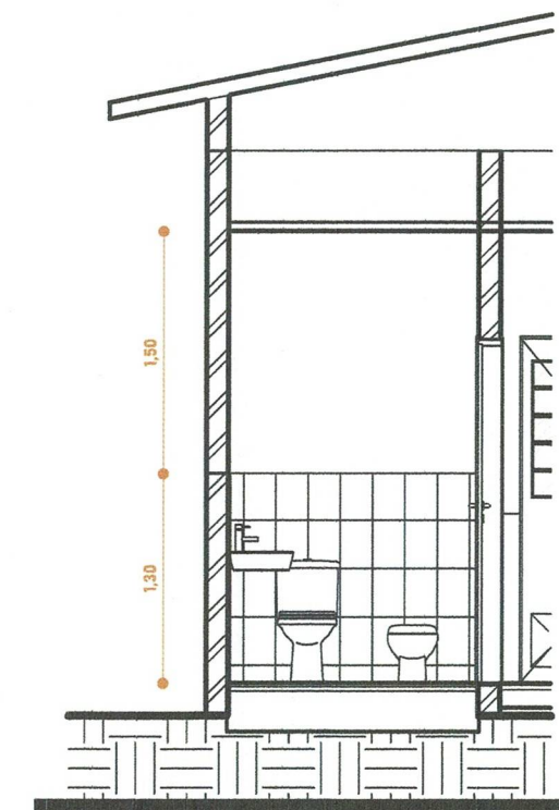
3 Corte 1 1:50
