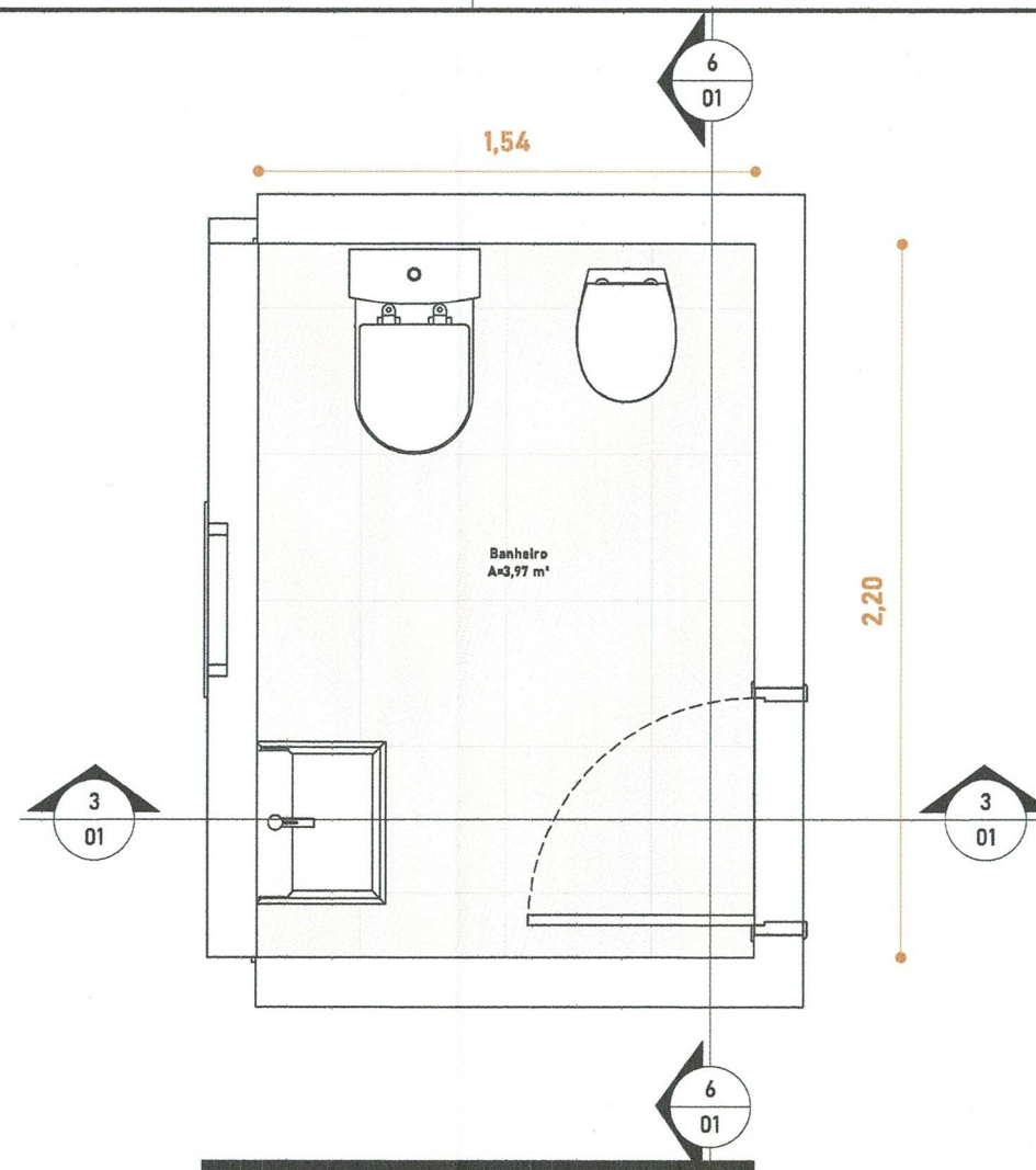
2 Banheiro 2 1:25
