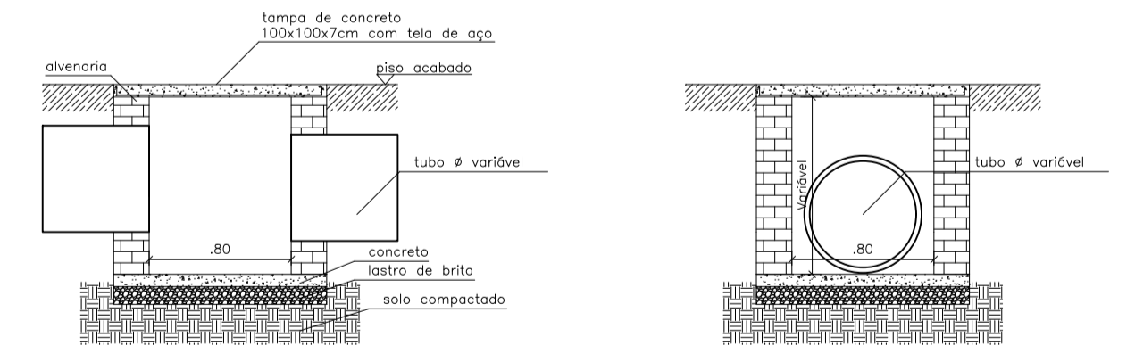
Detalhe Caixa de Passagem Sem Escala
