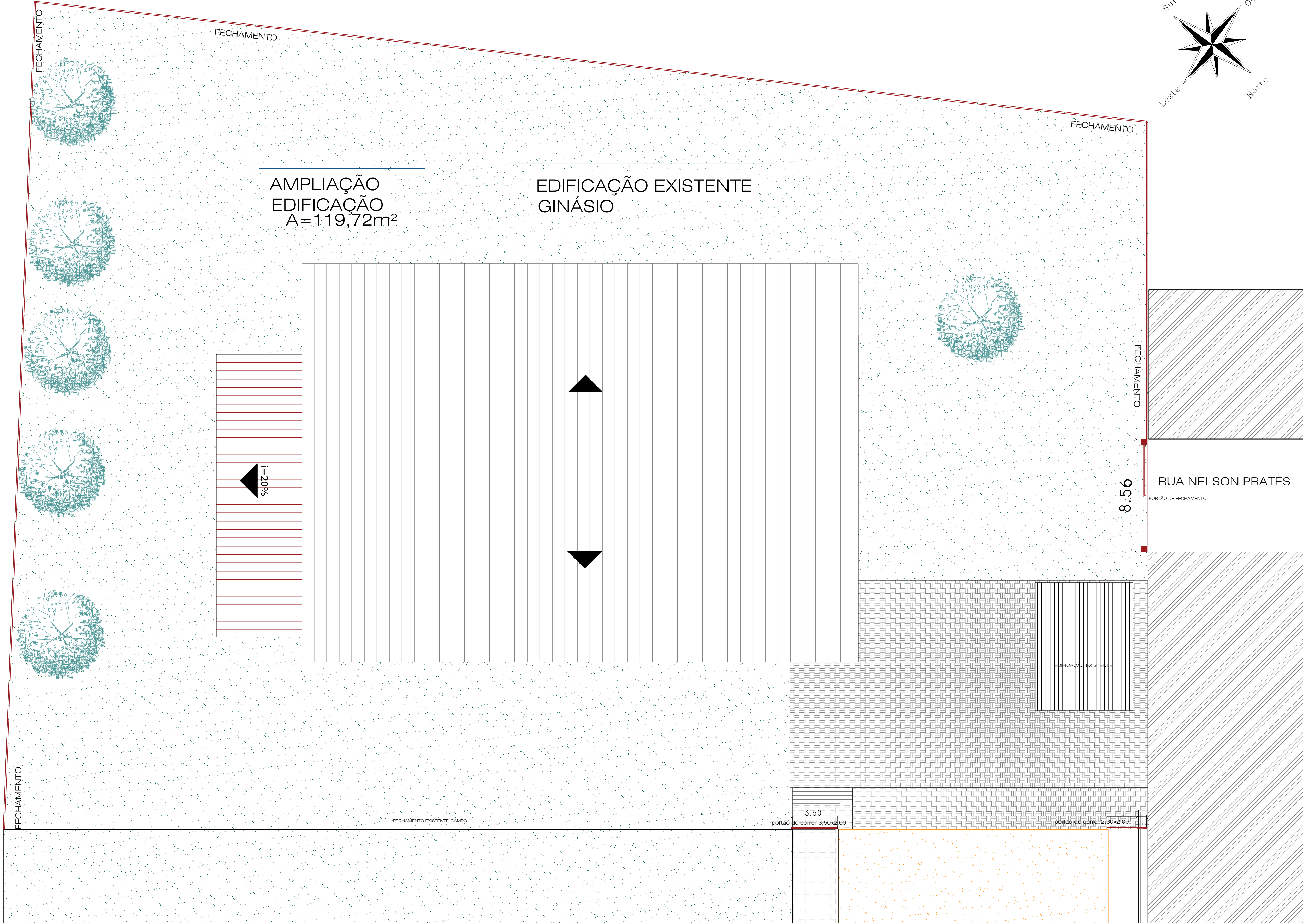
02 Planta de Situação ESCALA 1:150
