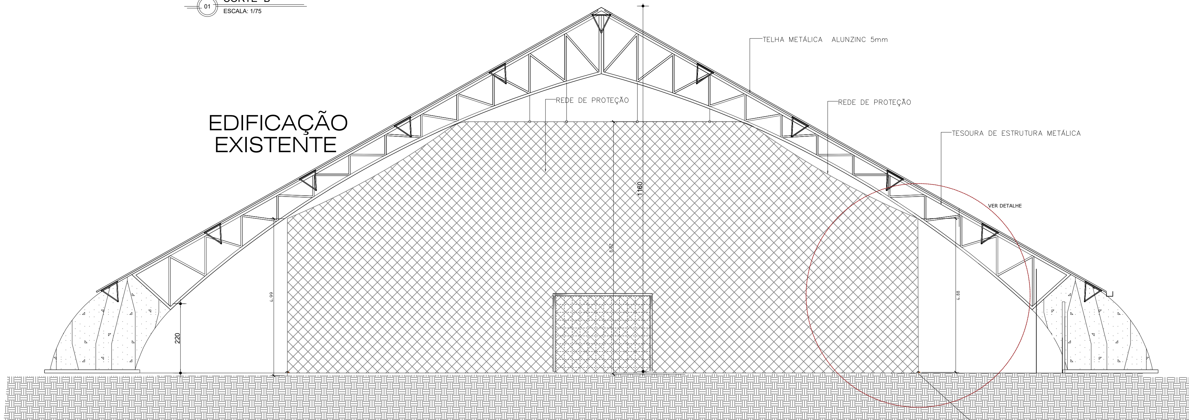
02 CORTE "C" ESCALA: 1/75
