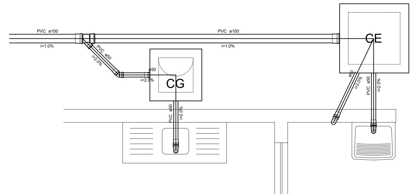
Detalhe Cozinha/Lavanderia escala 1:25
