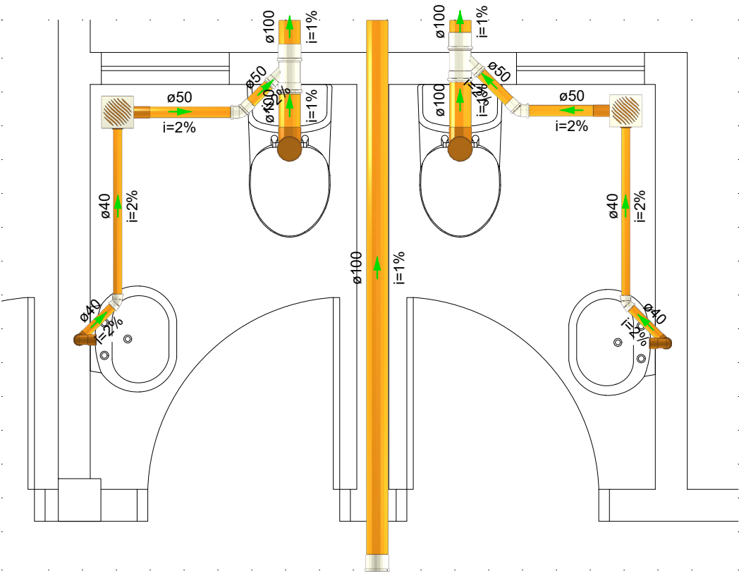
DETALHE WC PÚBLICO
