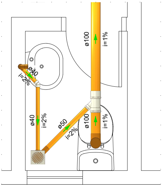
DETALHE WC SECRETÁRIA
