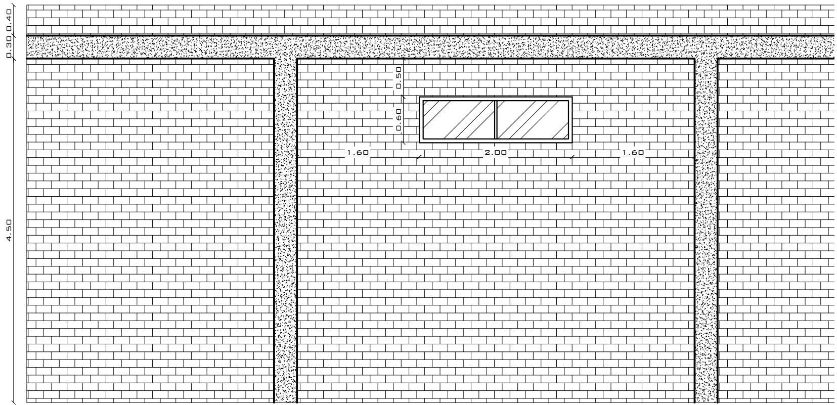
DETALHE PAREDES PAVILHÃO ESCALA 1:50
