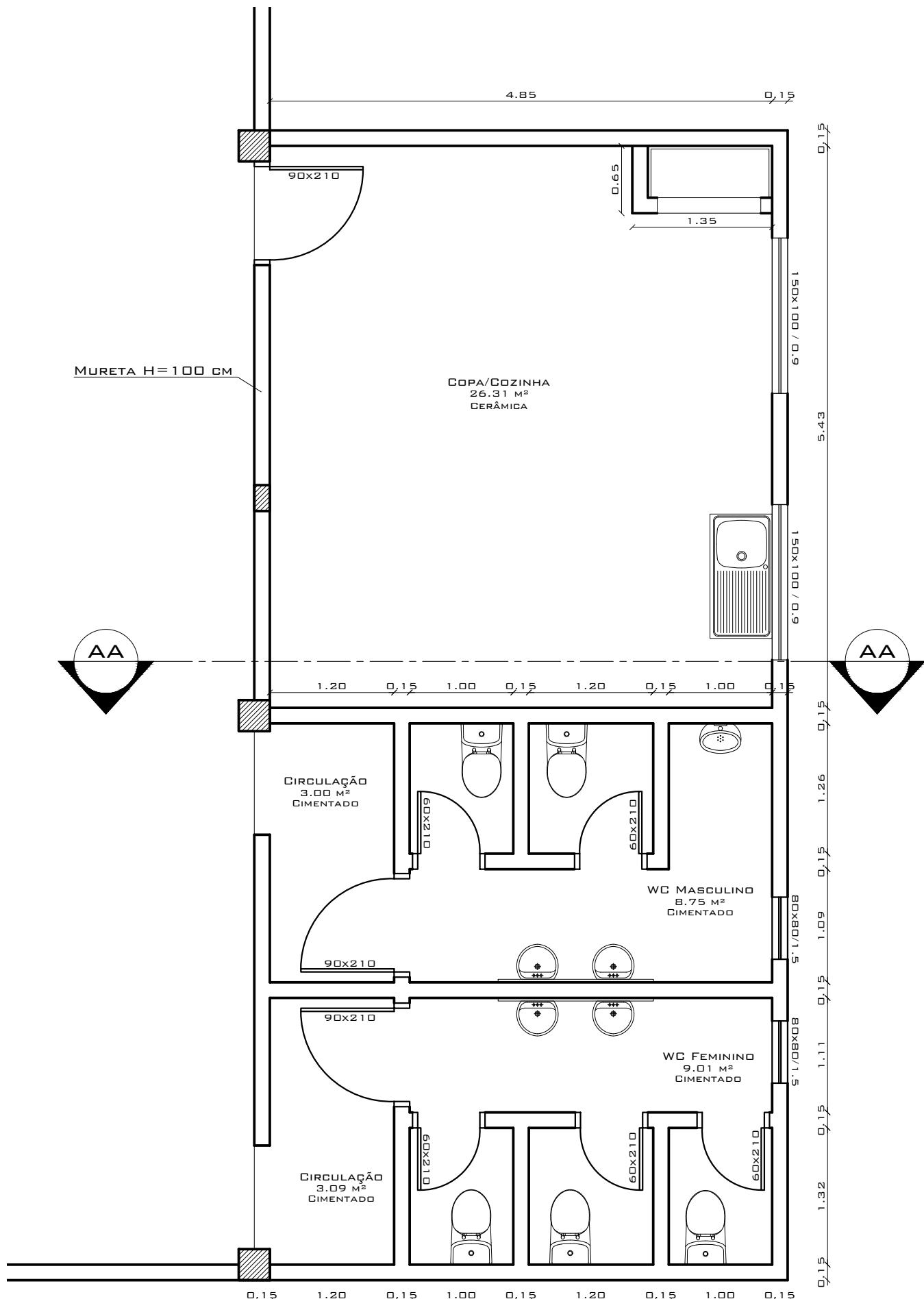
PLANTA BAIXA SANITÁRIOS E COPA ESCALA 1:50
