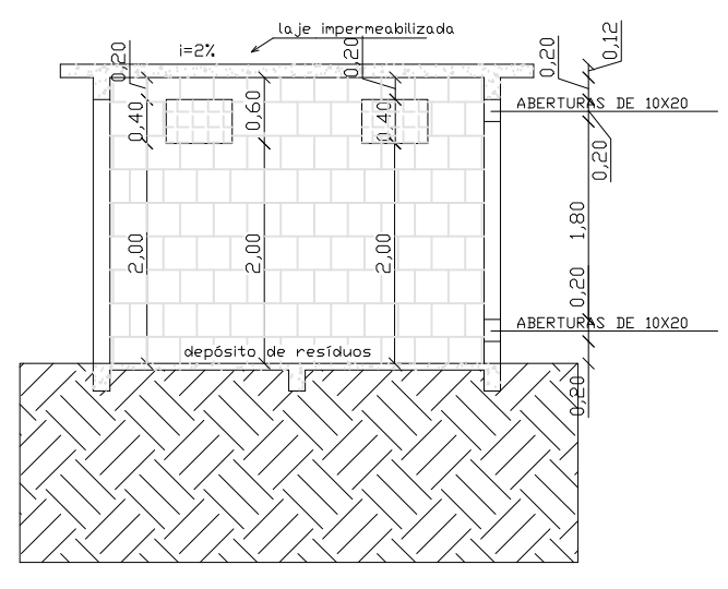
CORTE E-F ESC. 1/50
