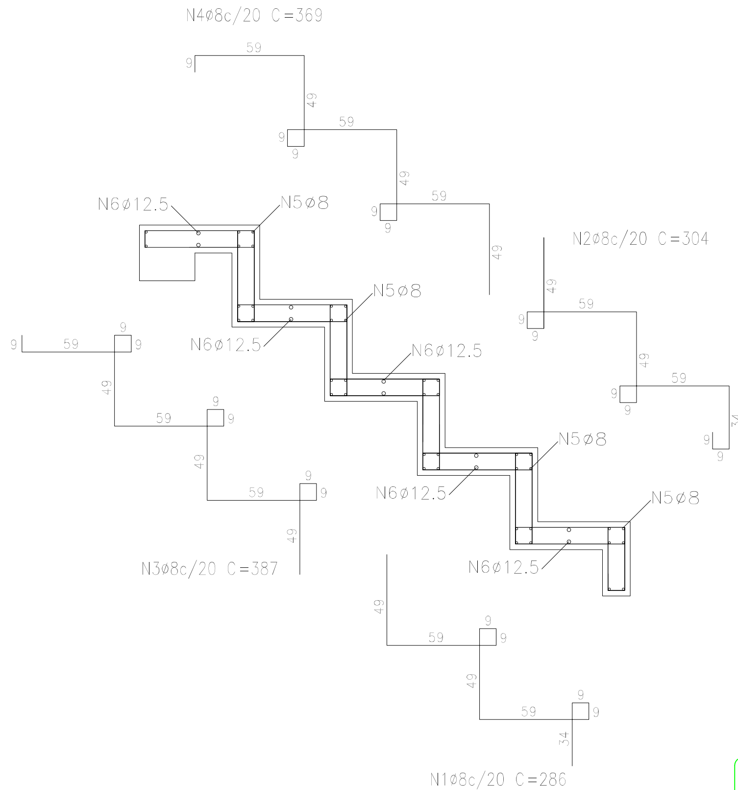
DETALHAMENTO ESTRUTURA esc. 1/20
