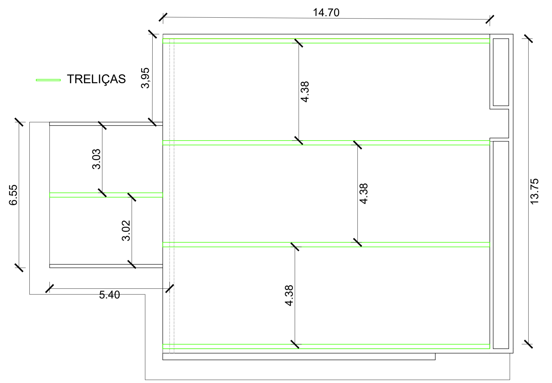
PLANTA DE DIMENSIONAMENTO DAS TRELIÇAS Escala: 1/100
