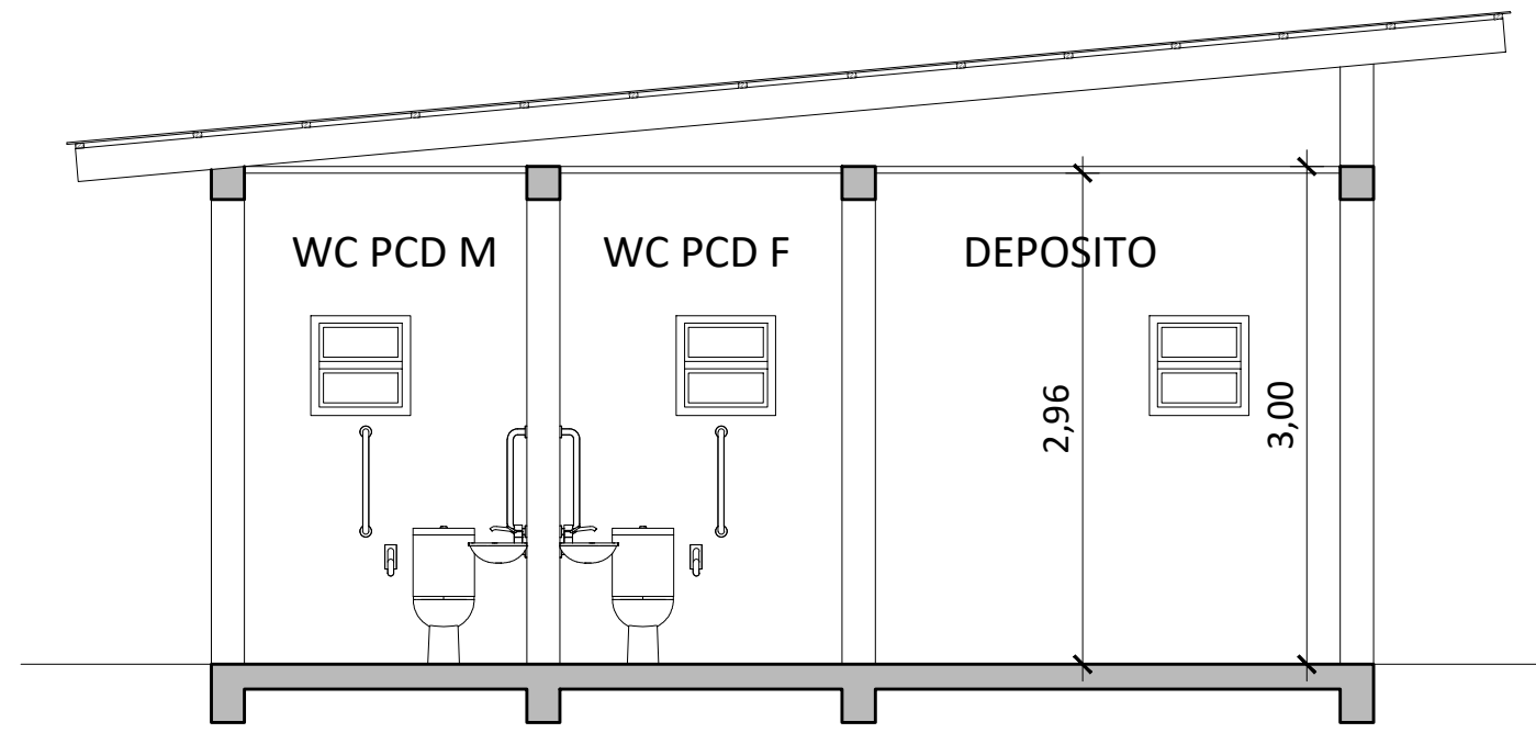
CORTE AA
