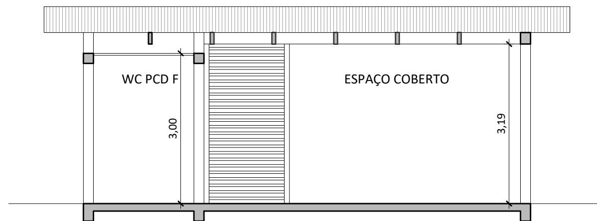
CORTE BB
