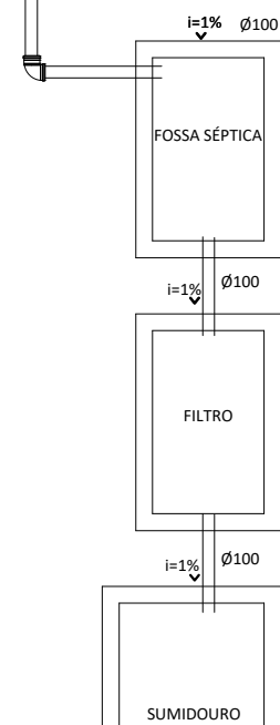
PLANTA BAIXA HIDROSSANITÁRIOS - ESGOTO
