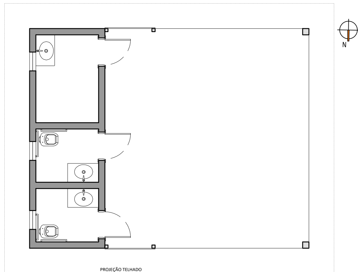
PLANTA BAIXA MOBILIADA
