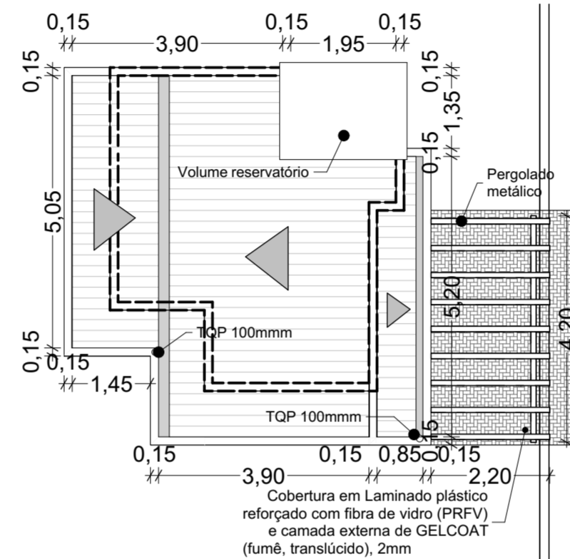
1. Planta de Cobertura Escala: 1:100
