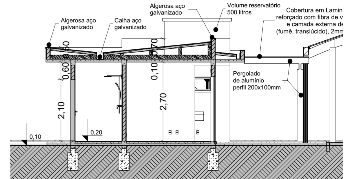
BB. Corte A - A Escala: 1:75
