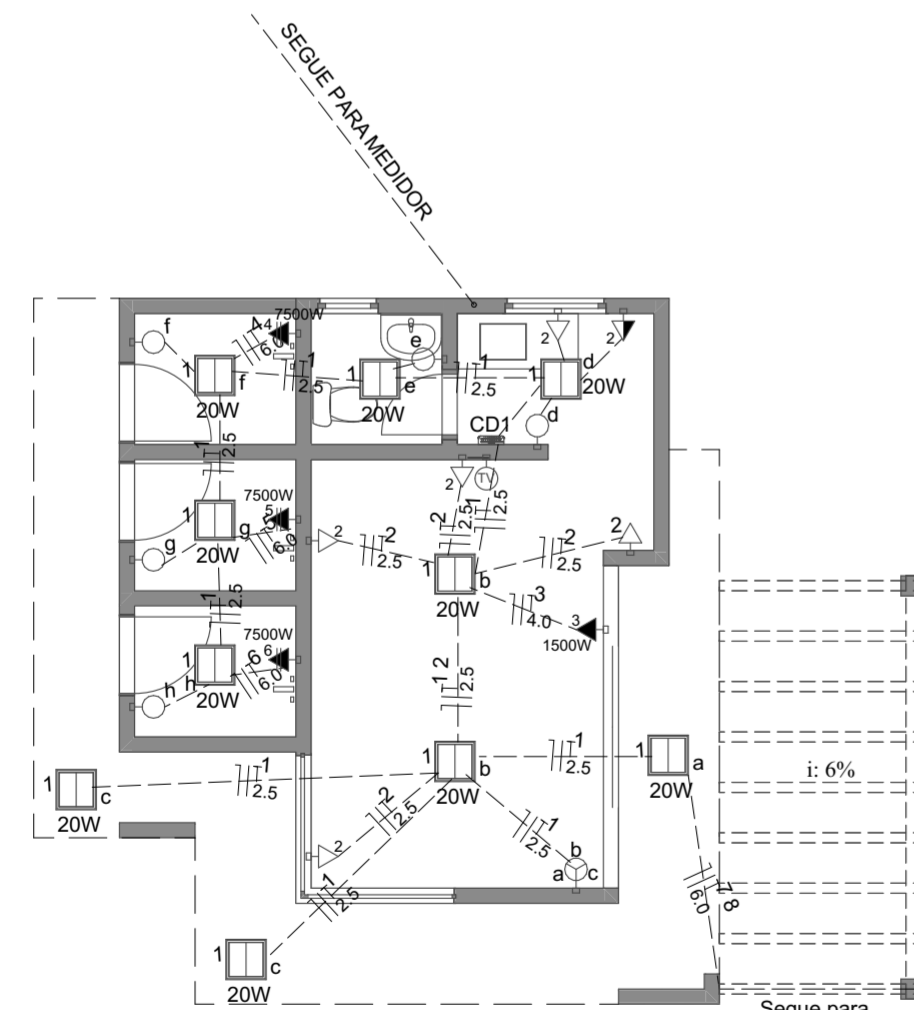
4. Instalações Elétricas Escala: 1:75
