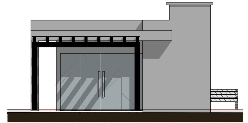
2. Fachada Oeste Escala: 1:75
