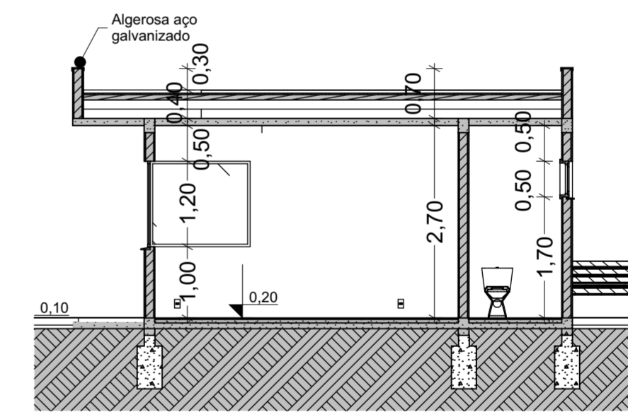
AA. Corte A - A Escala: 1:75
