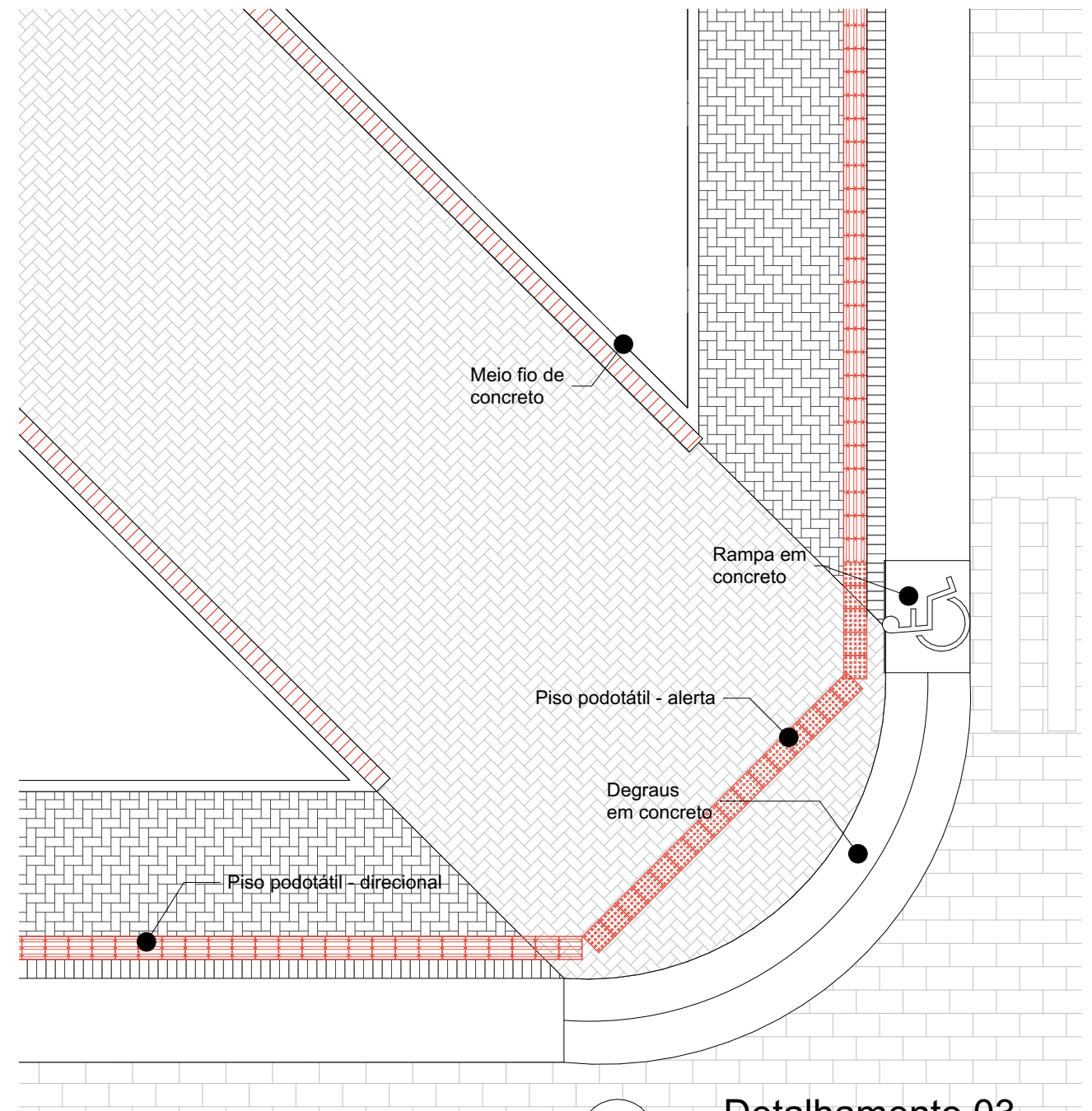
03 Detalhamento 03 Escala: 1:100
