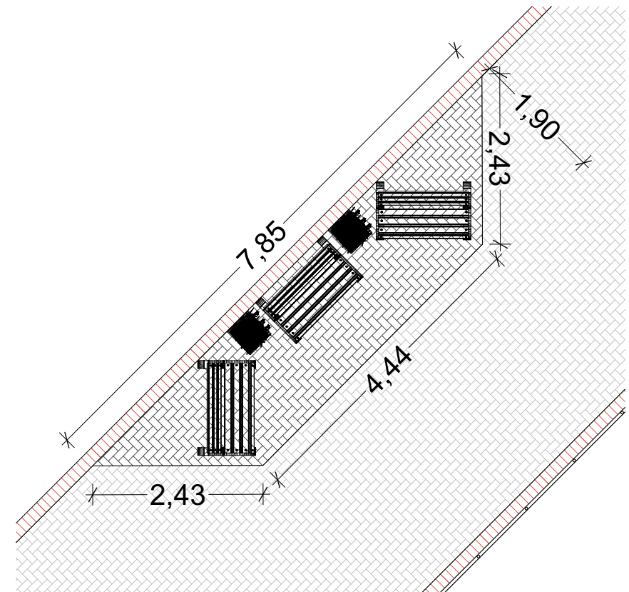
02 Detalhamento 02 Escala: 1:100
