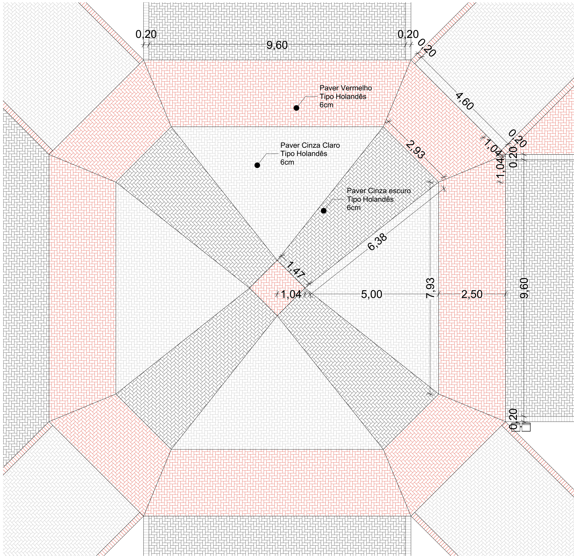
01 Detalhamento 01 Escala: 1:100
