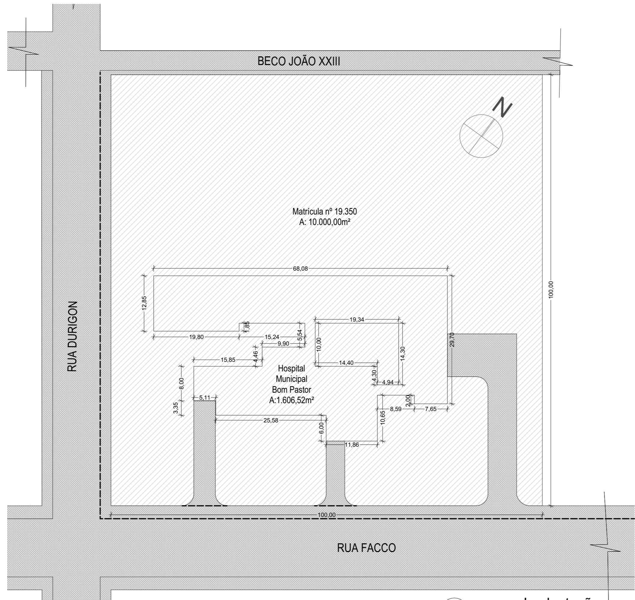
1 Implantação Escala: 1:500
