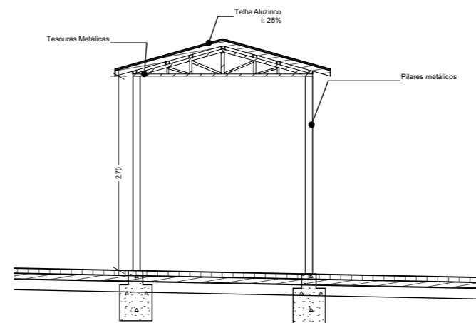
A Corte A - A Escala: 1:75
