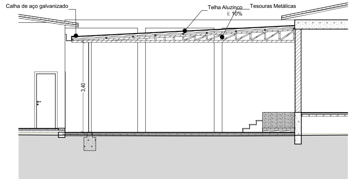
B Corte B - B Escala: 1:75
