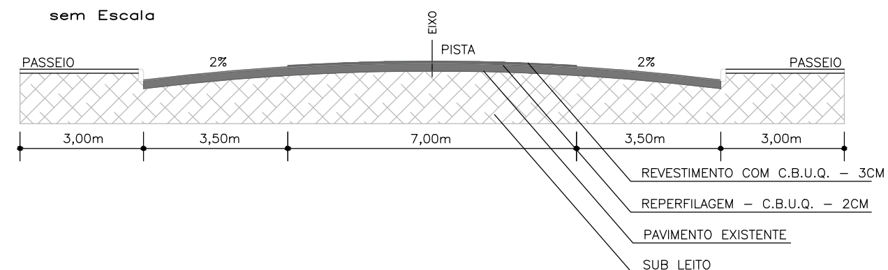
Corte Esquemático Transversal RUA RUBERT sem Escala
