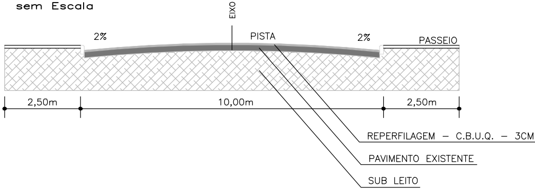
Corte Esquemático Transversal RUA ROSA sem Escala
