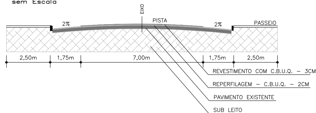
Corte Esquemático Transversal RUA JÂNIO QUADROS sem Escala
