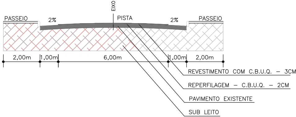
Corte Esquemático Transversal RUA DOS GUARANIS sem Escala
