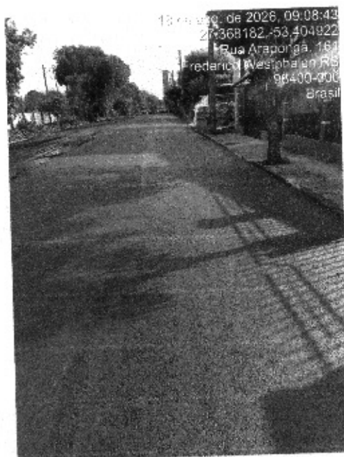
Foto 05 – Pavimentação.
