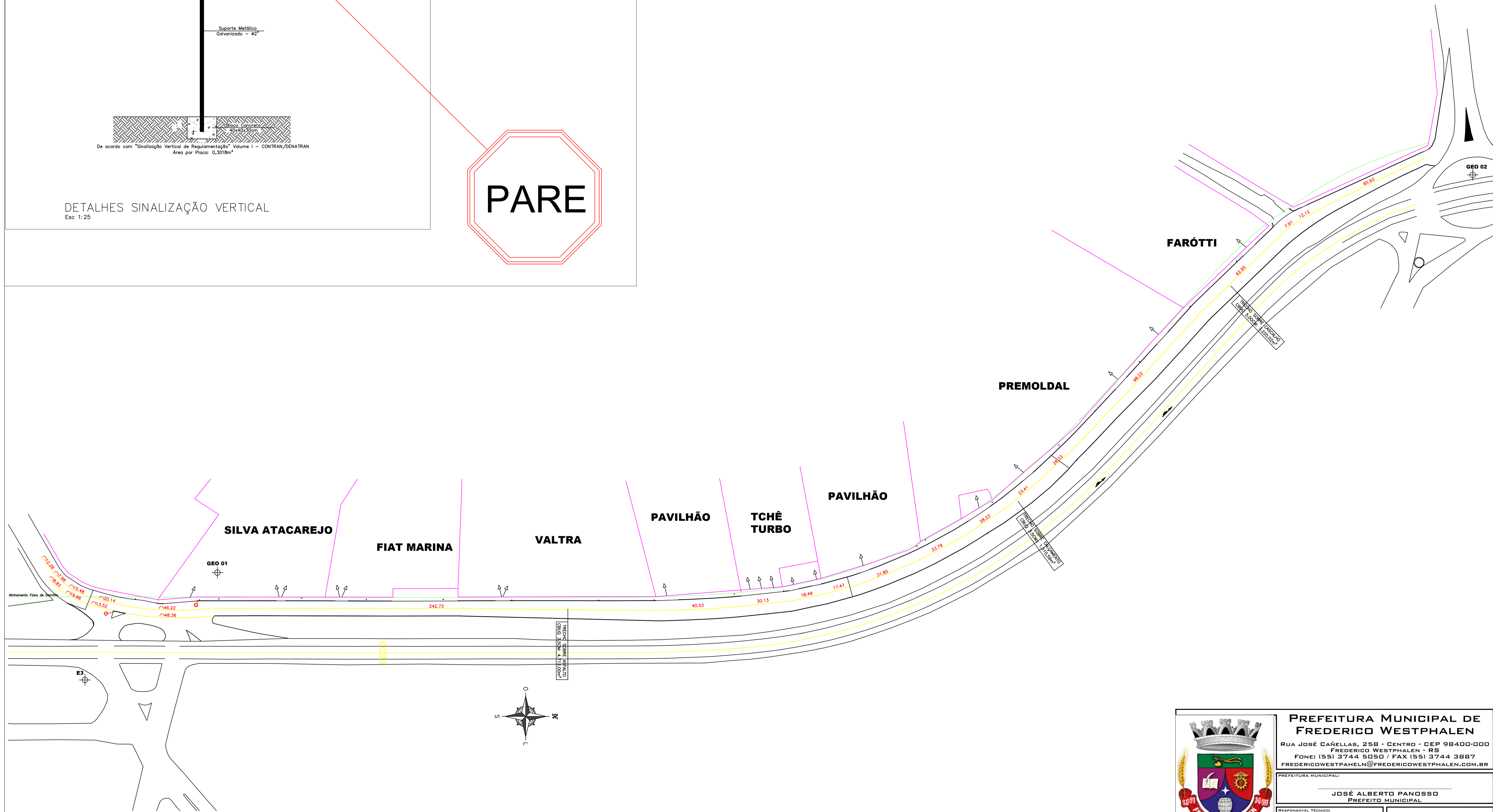
PLANTA SINALIZAÇÃO Esc 1:1000
