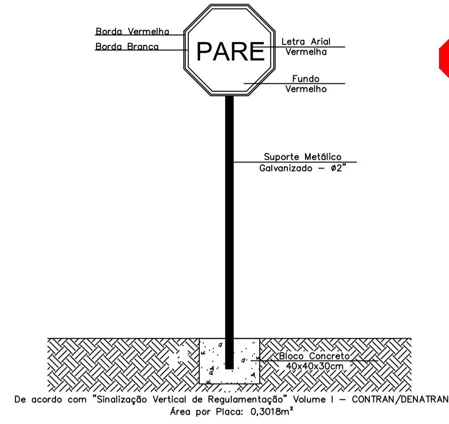
DETALHES SINALIZAÇÃO VERTICAL Esc 1:25
