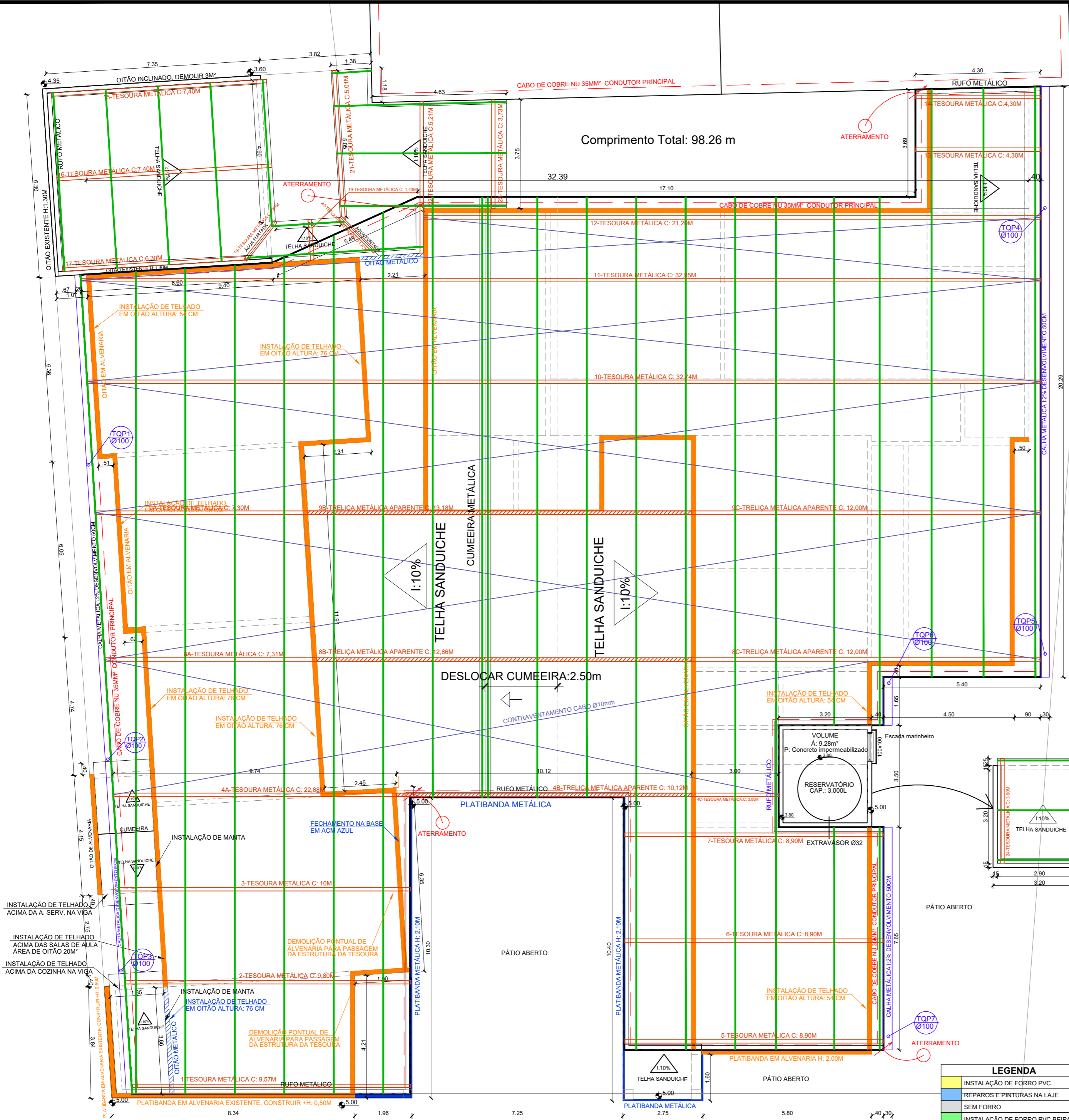
05 PLANTA DE COBERTURA ESCALA 1/100 ÁREA: 111M²
