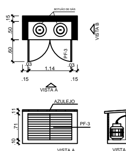
DETALHE DE ESQUADRIAS
